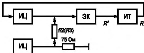
Рисунок 15 — Схема проверки устойчивости ЦРЛТ к составному сигналу
