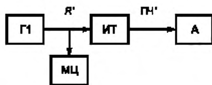
Рисунок 19 — Схема измерения девиации несущей частоты, вызванной сигналом основной полосы, и девиации несущей частоты, вызванной пилот-сигналом
