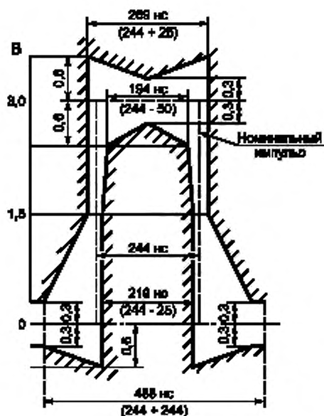
Рисунок 3 — Маска импульса на стыке 2,048 Мбит/с
