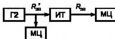
Рисунок 26 — Схема измерения уровней сигнала в канале звука
