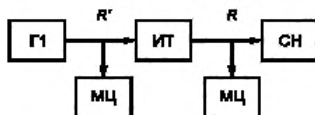
Рисунок 18 — Схема измерения номинальных уровней сигнала и основной полосы частот линейного тракта
