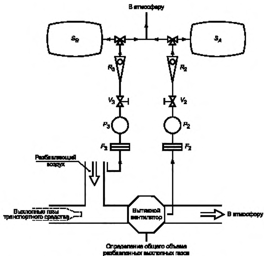
ПРИМЕР 1. Оборудование для отбора проб газа и измерения объема
