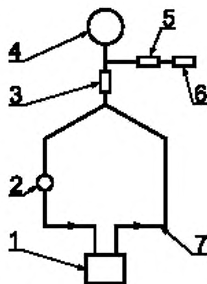
1 — аппарат ИВЛ; 2 — проверяемое устройство для измерения объема; 3 — сопротивление; 4 — модель легких; 5 — датчик давления; 6 — регистратор давления с предельной погрешностью \pm 2\% действительного значения для проверки точности устройства измерения объема; 7 — дыхательный контур
