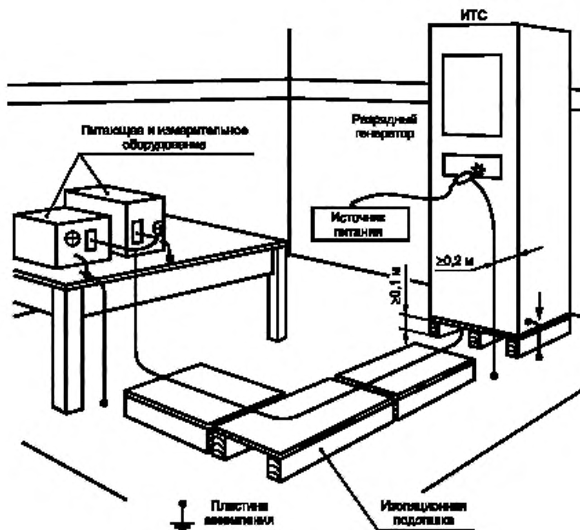
Рисунок 3 — Пример рабочего места для испытаний
