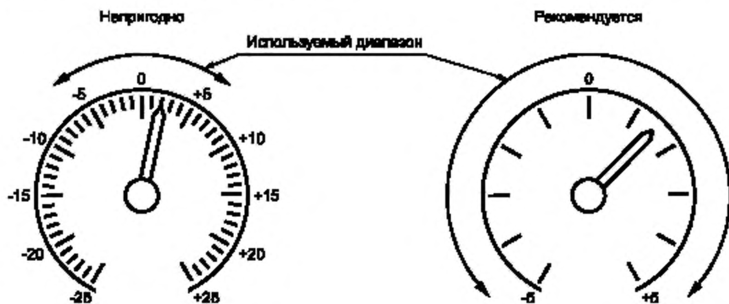
Рисунок 7 — Правильное и неправильное применение шкал
