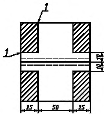
1 – линия разреза
