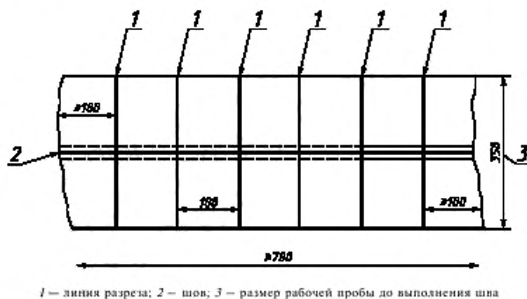
Рисунок 1 — Проба со швом и разметкой для изготовления точечных проб
