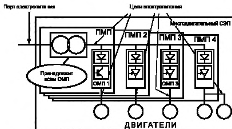
Рисунок 4 — Цепи электропитания СЭП с общим входным трансформатором
