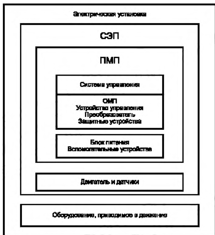
Рисунок 1 — Составные части электрической установки, включающей СЭП
