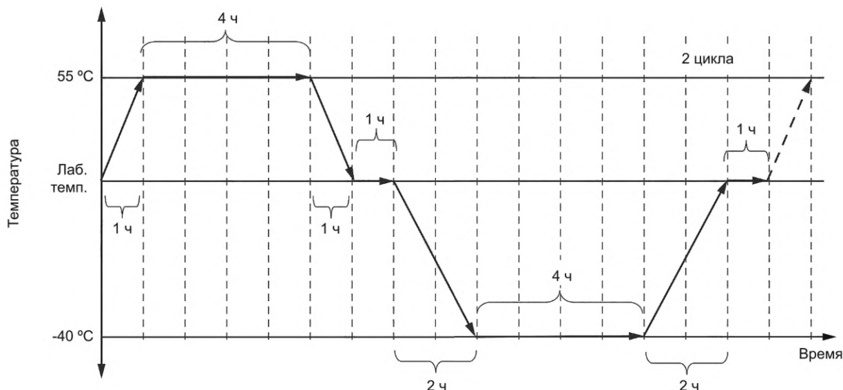
Рисунок 3 — Температурный профиль одного цикла проведения испытания на циклическое изменение температур (термоциклирование)
