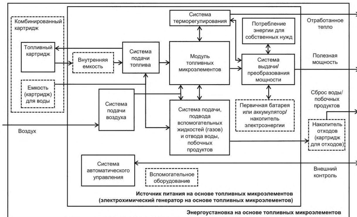
Рисунок 1 — Блок-схема энергоустановки на основе топливных микрэлементов
