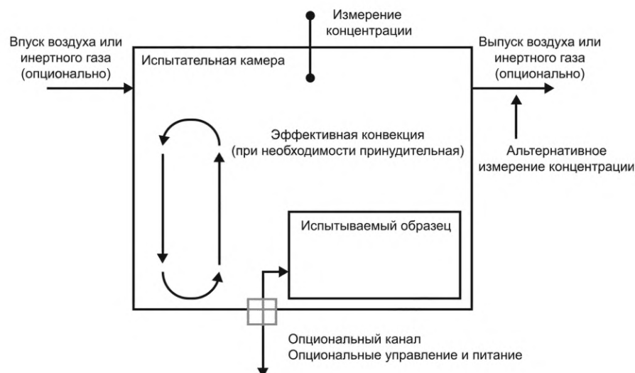
Рисунок 4 — Оборудование для проведения измерений выбросов газов
