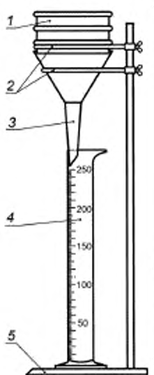
1 — сито; 2 — кольцо; 3 — стеклянная воронка; 4 — мерный цилиндр; 5 — штатив
