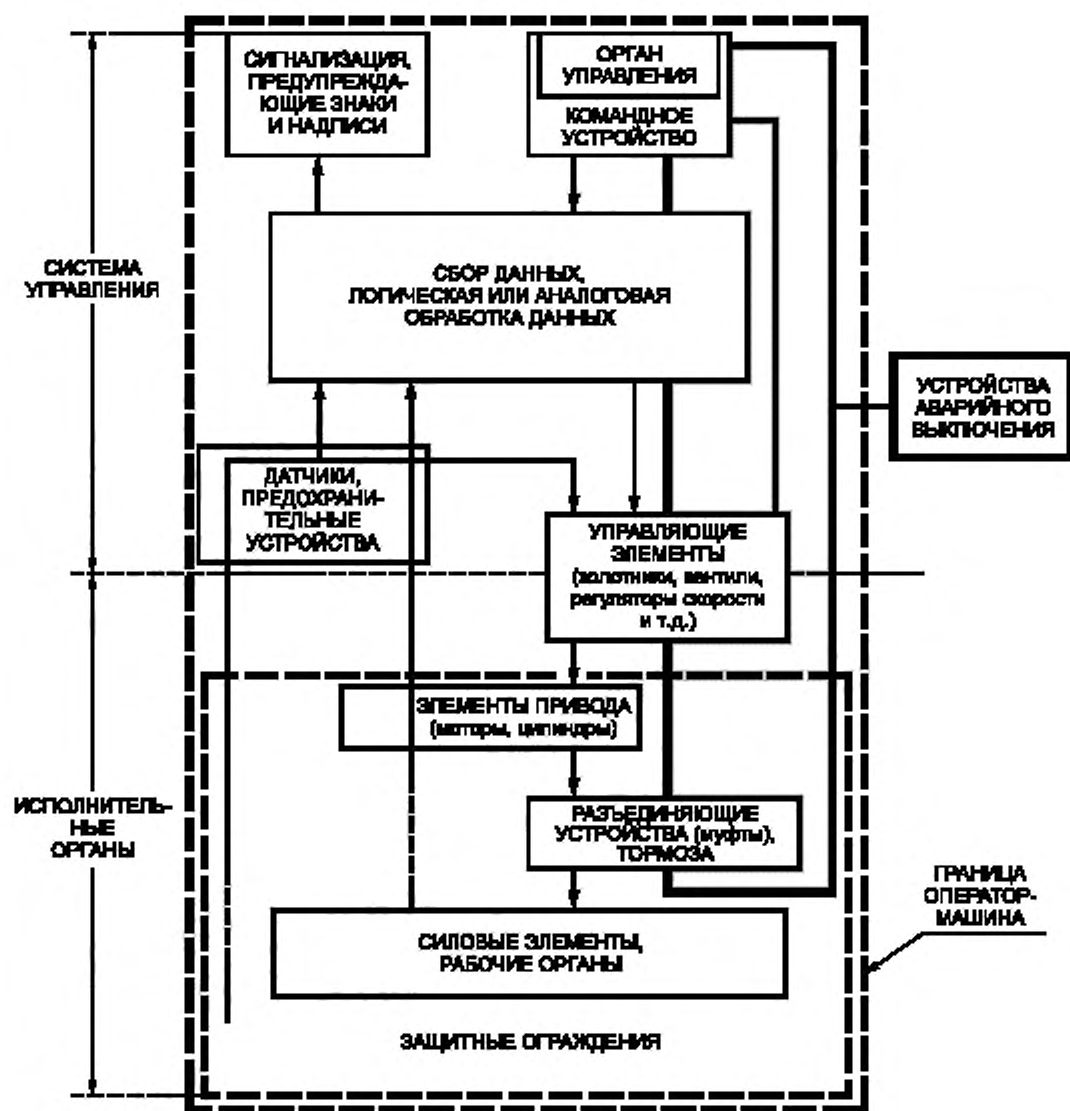
Рисунок 2 — Устройства аварийного отключения машины/сооружения
