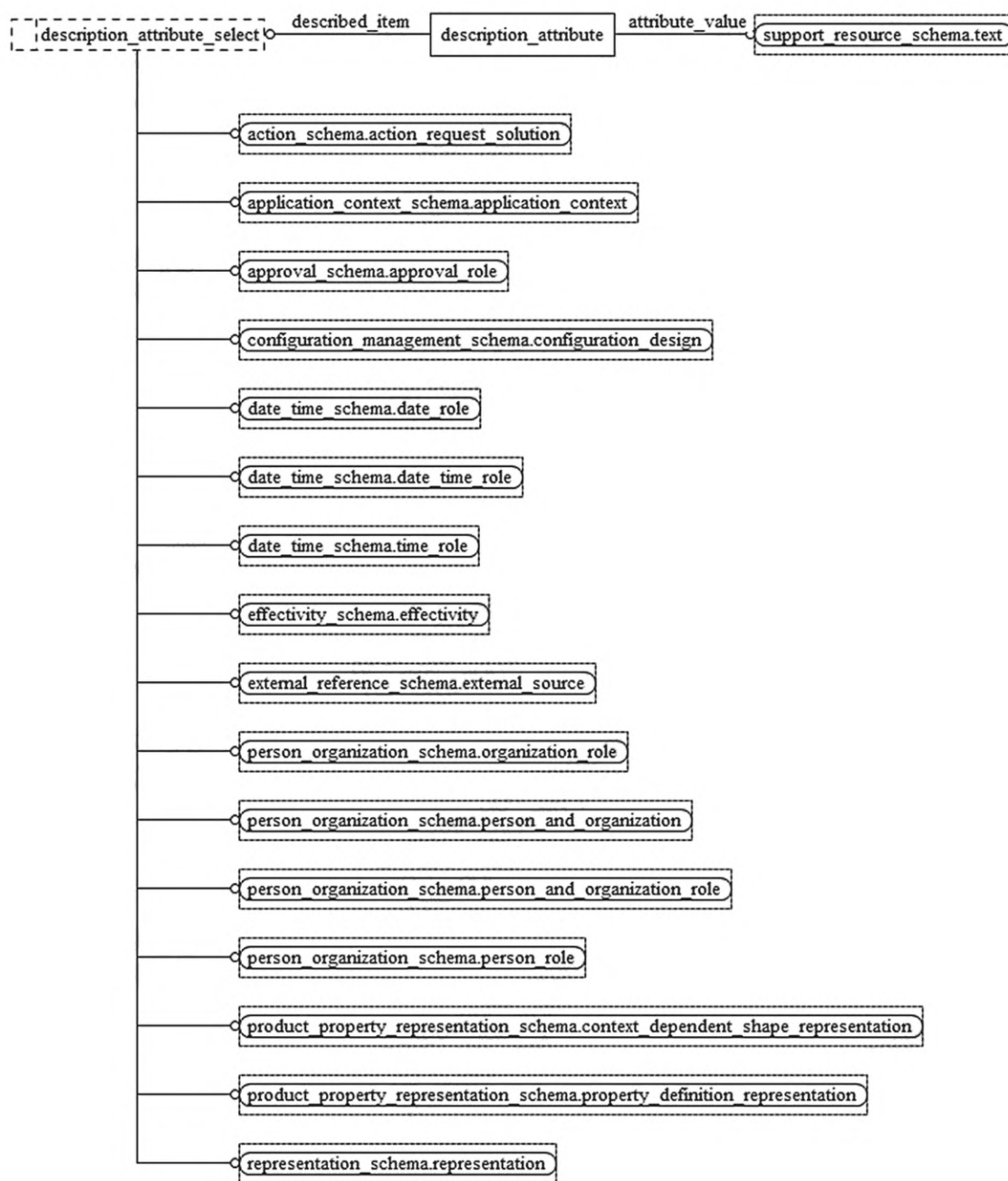
Рисунок D.9 — EXPRESS-G диаграмма схемы basic_attribute_schema (диаграмма 3 из 5)
