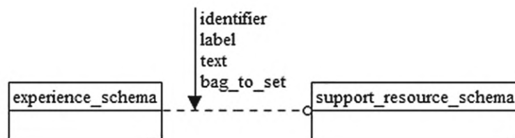
Рисунок D.23 — EXPRESS-G диаграмма схемы experience_schema (диаграмма 1 из 2)
