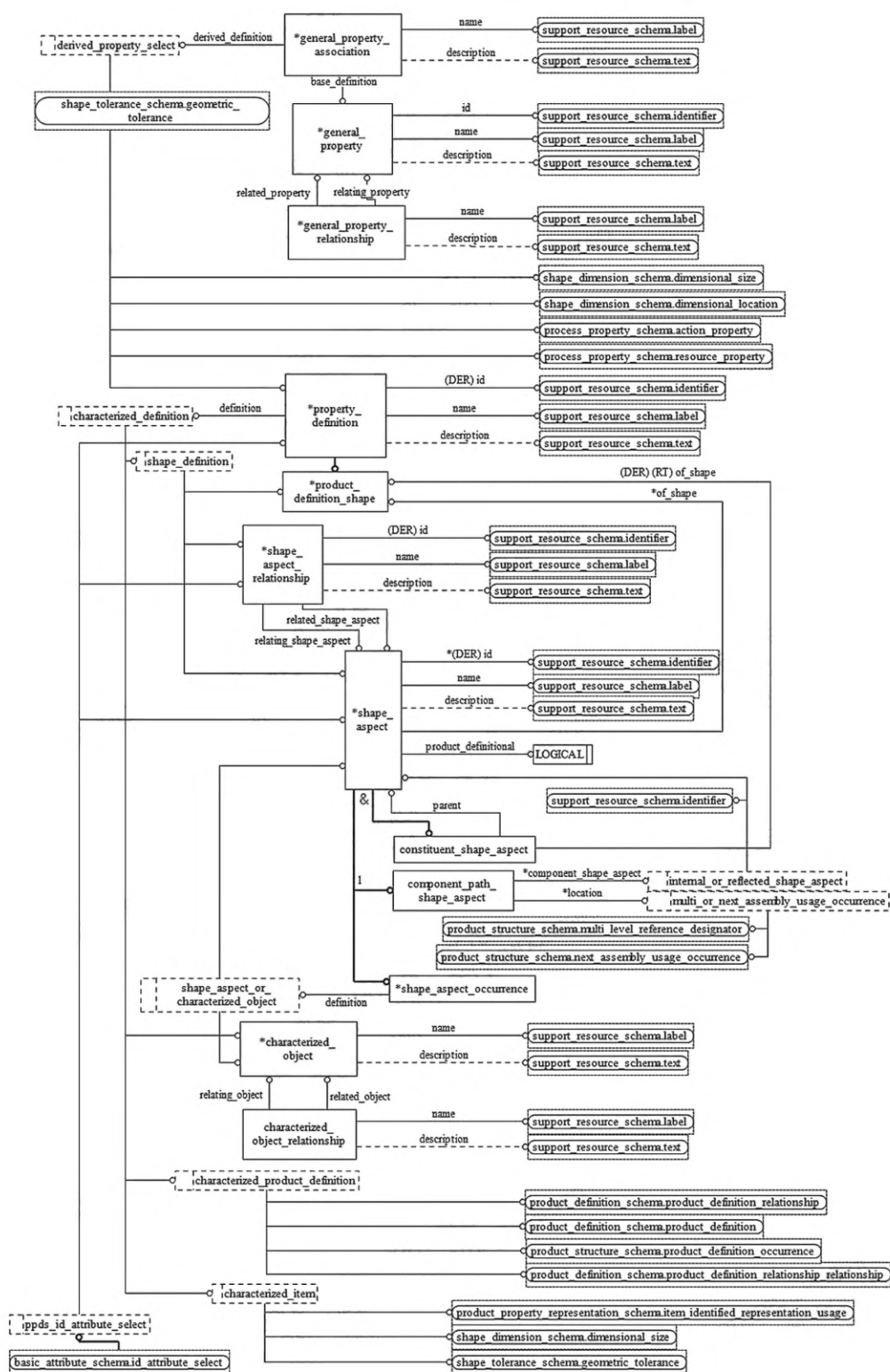
Рисунок D.55 — EXPRESS-G диаграмма схемы product_property_definition_schema (диаграмма 2 из 2)
