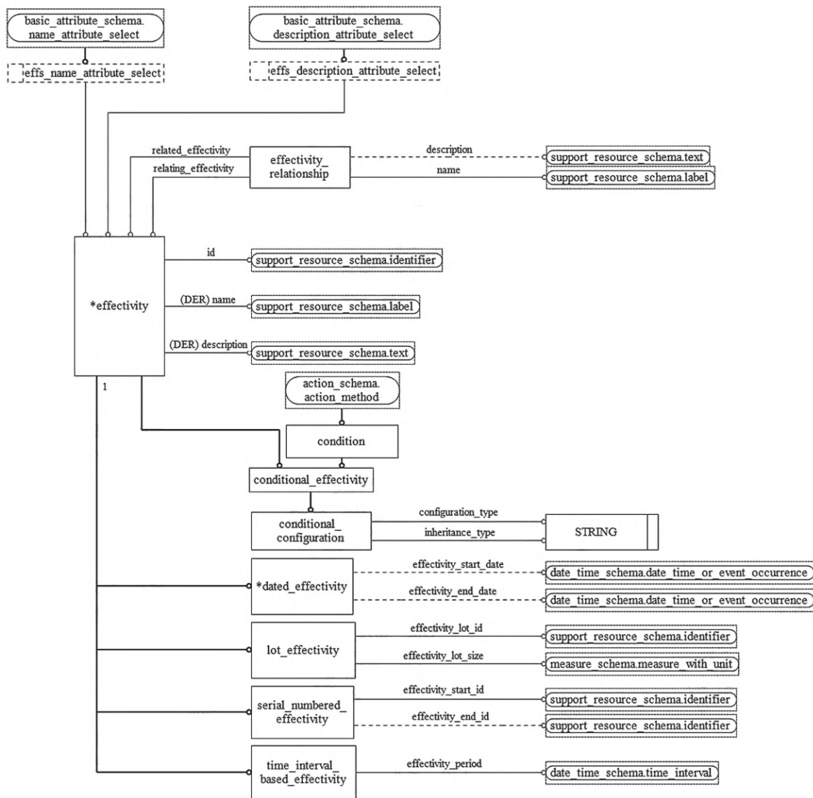
Рисунок D.22 — EXPRESS-G диаграмма схемы effectivity_schema (диаграмма 2 из 2)
