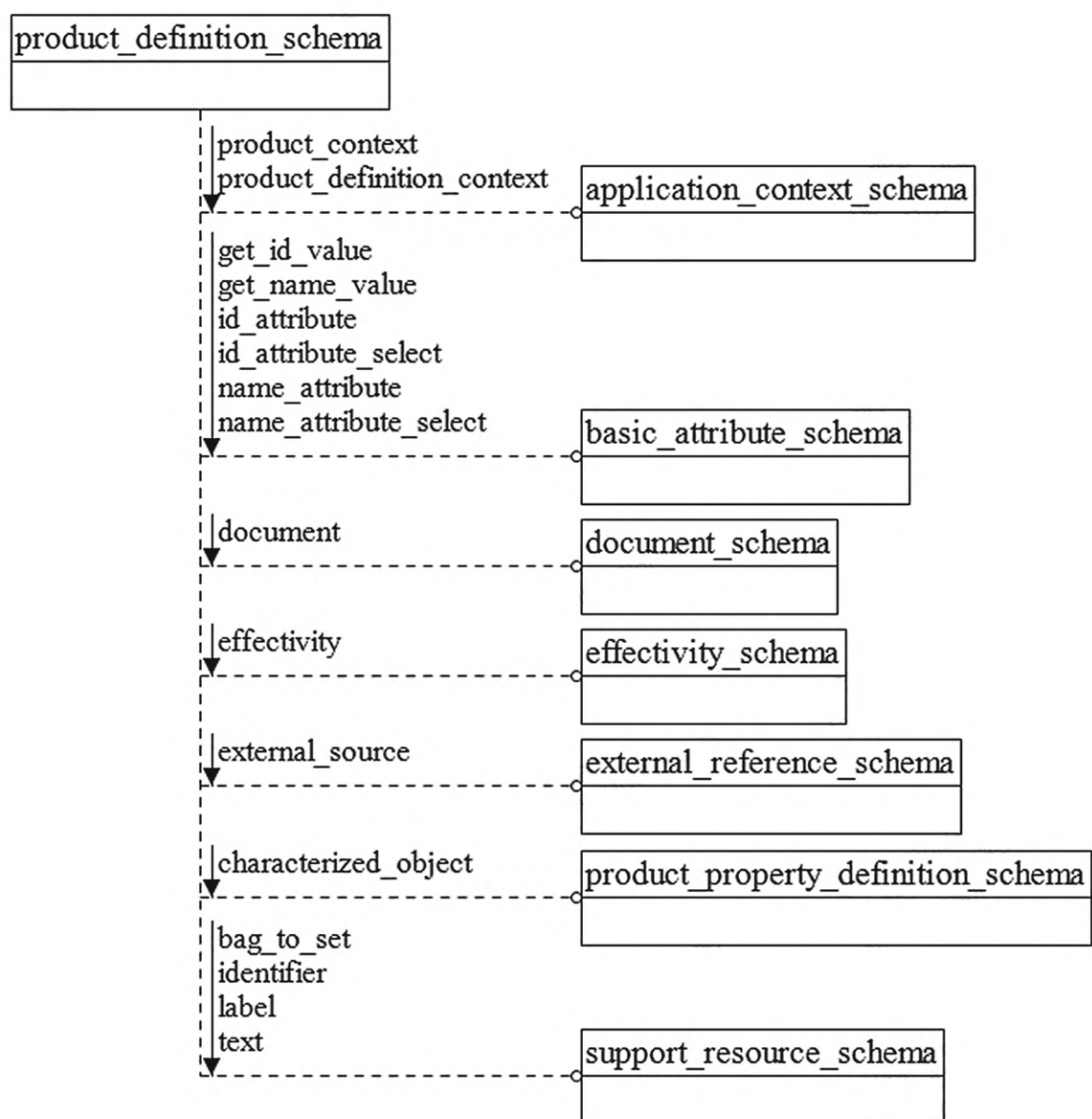
Рисунок D.51 — EXPRESS-G диаграмма схемы product_definition_schema (диаграмма 1 из 3)
