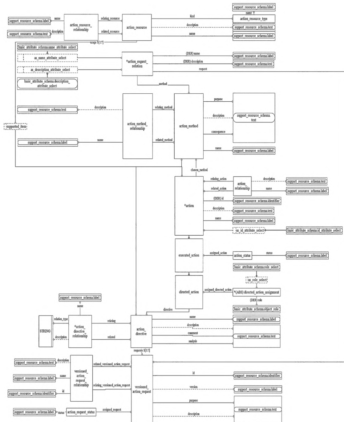
Рисунок D.2 — EXPRESS-G диаграмма схемы action_schema (диаграмма 2 из 2)
