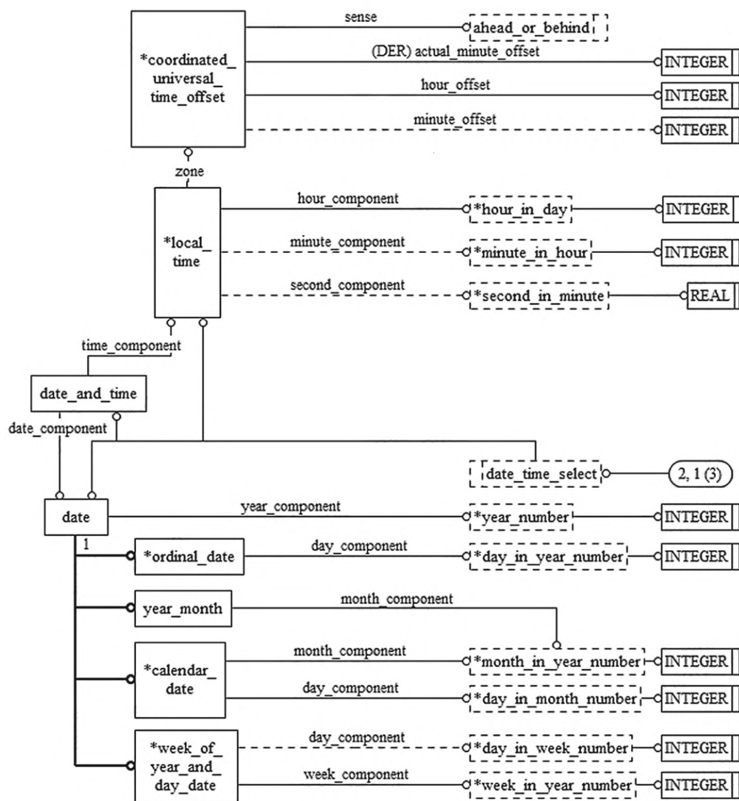
Рисунок D.17 — EXPRESS-G диаграмма схемы date_time_schema (диаграмма 2 из 3)
