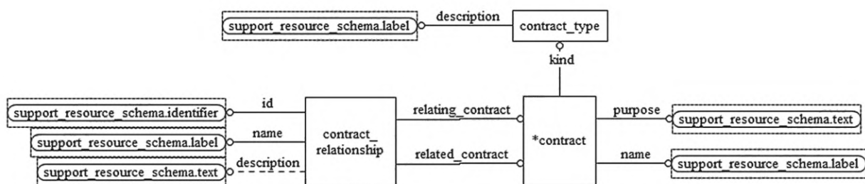
Рисунок D.15 — EXPRESS-G диаграмма схемы contract_schema (диаграмма 2 из 2)
