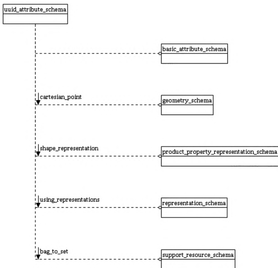
Рисунок D.64 — EXPRESS-G диаграмма схемы uuid_attribute_schema (диаграмма 1 из 2)
