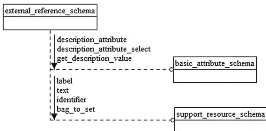
Рисунок D.25 — EXPRESS-G диаграмма схемы external_reference_schema (диаграмма 1 из 2)
