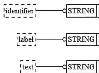
Рисунок D.63 — EXPRESS-G диаграмма схемы support_resource_schema (диаграмма 2 из 2)
