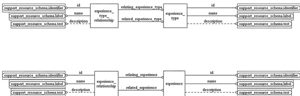
Рисунок D.24 — EXPRESS-G диаграмма схемы experience_schema (диаграмма 2 из 2)
