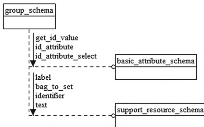
Рисунок D.27 — EXPRESS-G диаграмма схемы group_schema (диаграмма 1 из 2)
