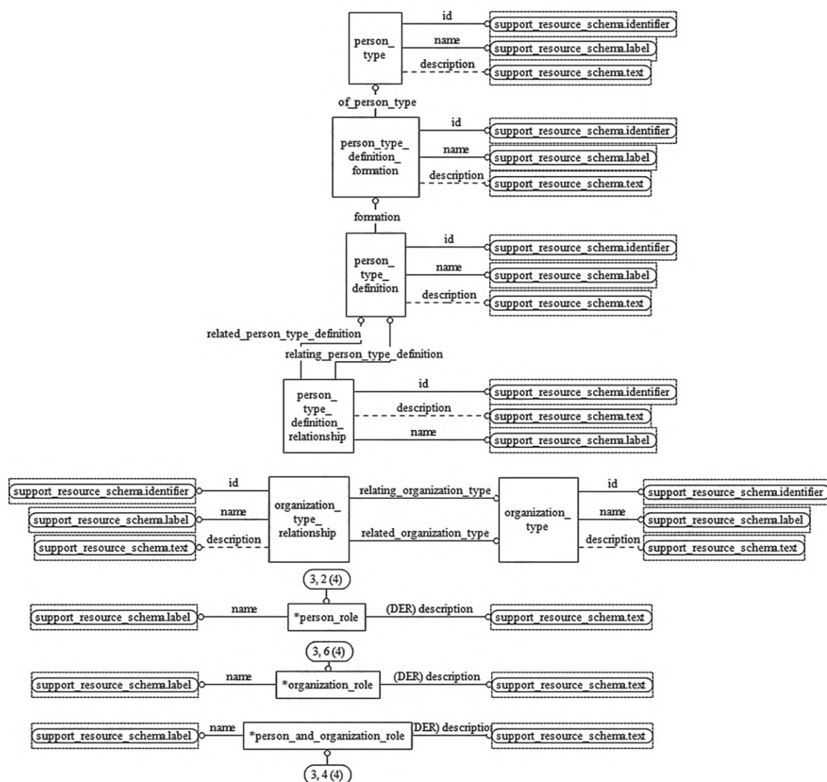
Рисунок D.49 — EXPRESS-G диаграмма схемы person_organization_schema (диаграмма 3 из 4)
