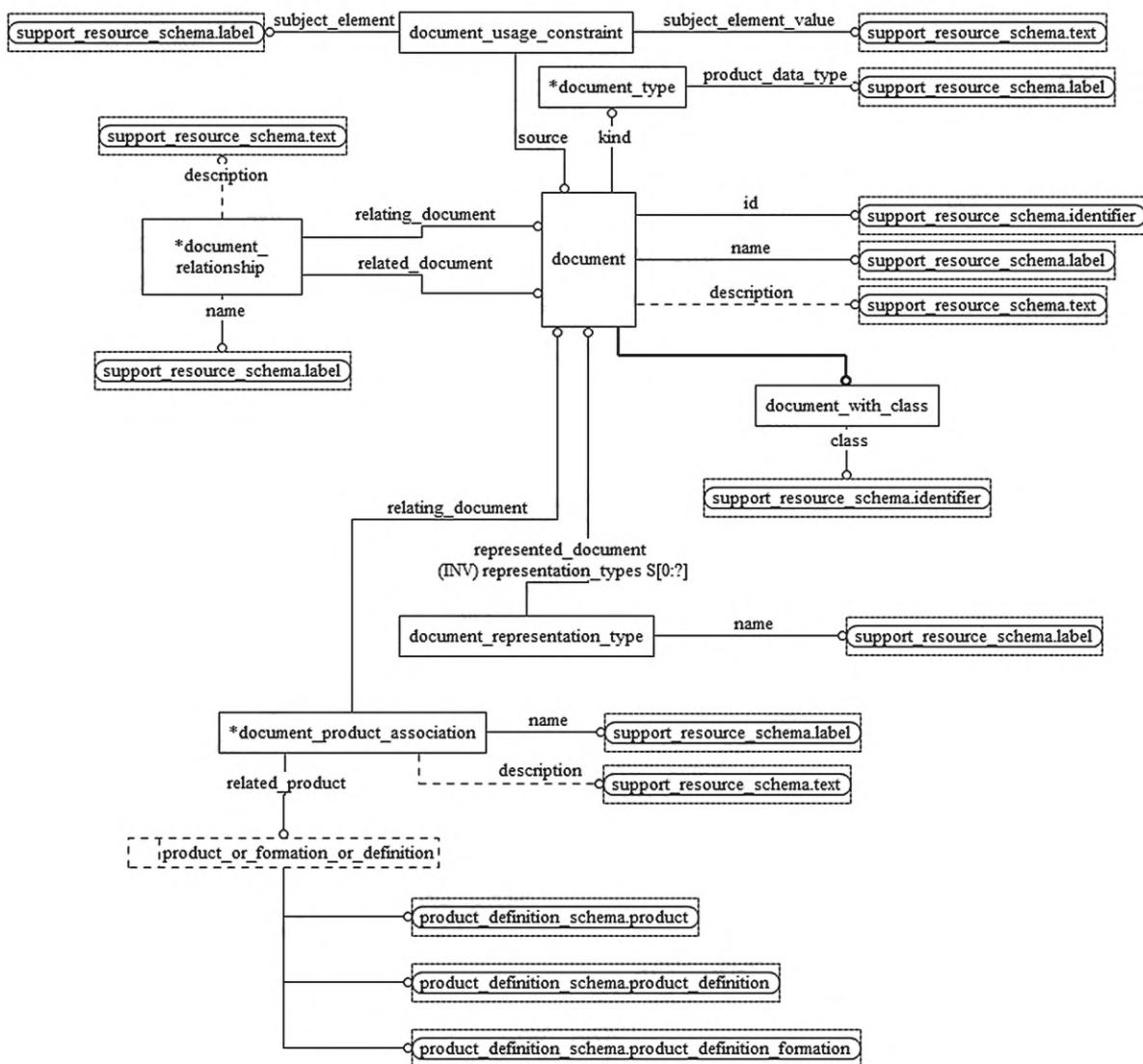
Рисунок D.20 — EXPRESS-G диаграмма схемы document_schema (диаграмма 2 из 2)
