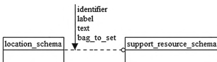
Рисунок D.31 — EXPRESS-G диаграмма схемы location_schema (диаграмма 1 из 2)
