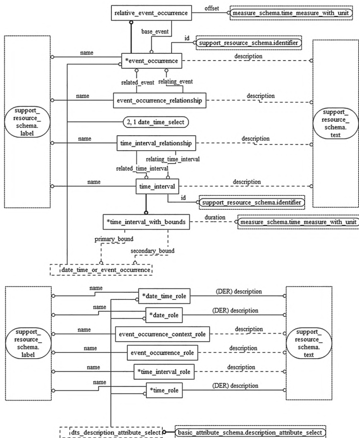
Рисунок D.18 — EXPRESS-G диаграмма схемы date_time_schema (диаграмма 3 из 3)
