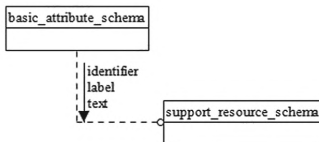
Рисунок D.7 — EXPRESS-G диаграмма схемы basic_attribute_schema (диаграмма 1 из 5)
