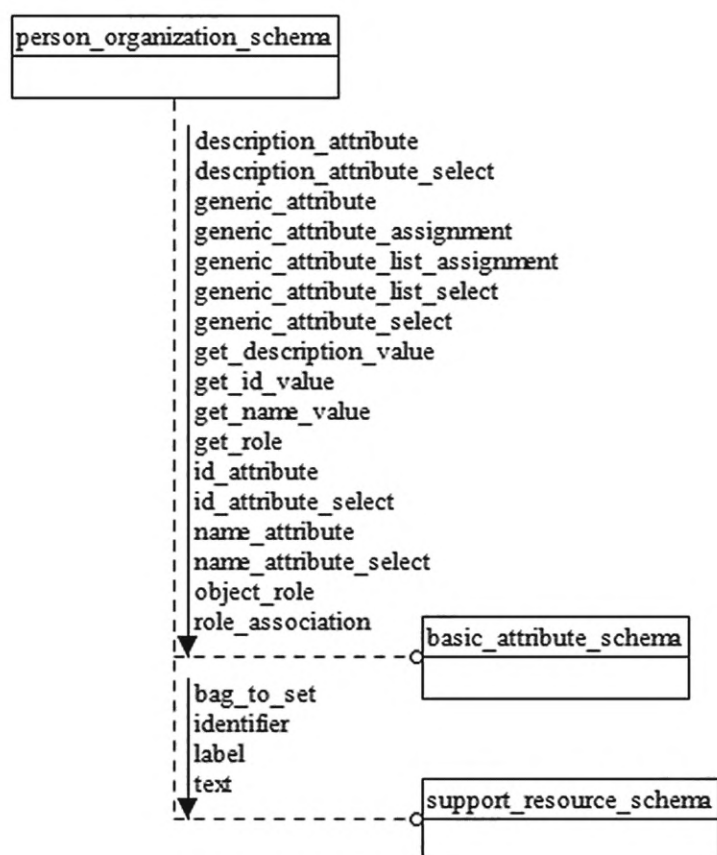
Рисунок D.47 — EXPRESS-G диаграмма схемы person_organization_schema (диаграмма 1 из 4)
