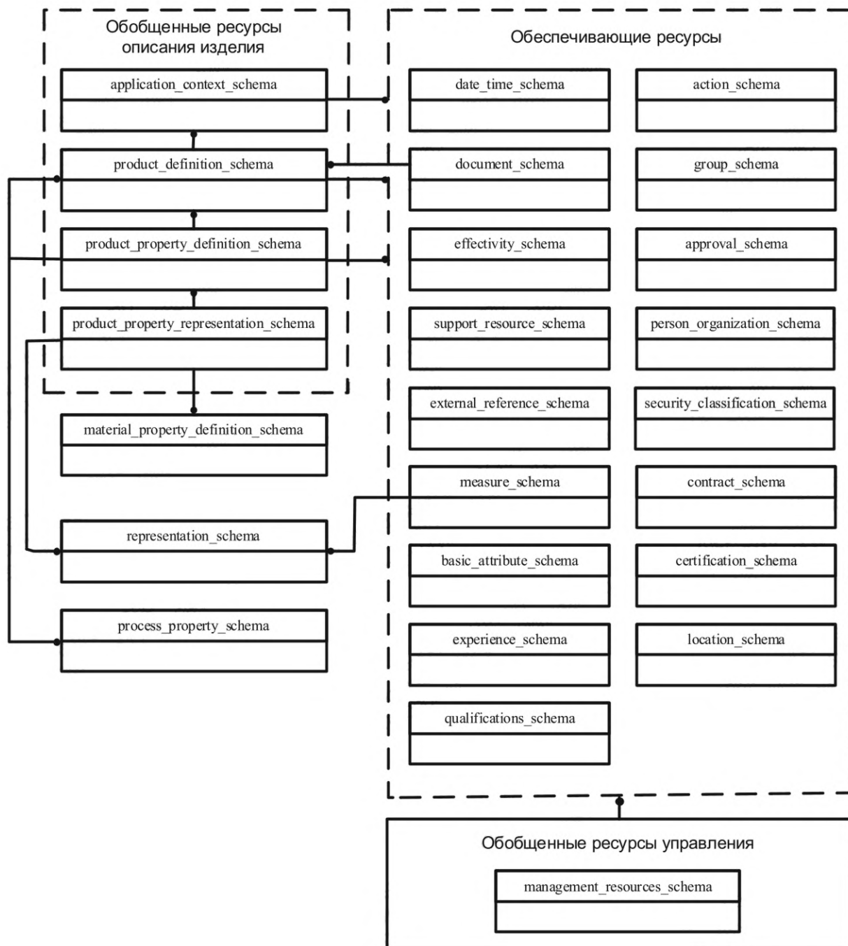
Рисунок 1 — Схемы, определенные в настоящем стандарте
