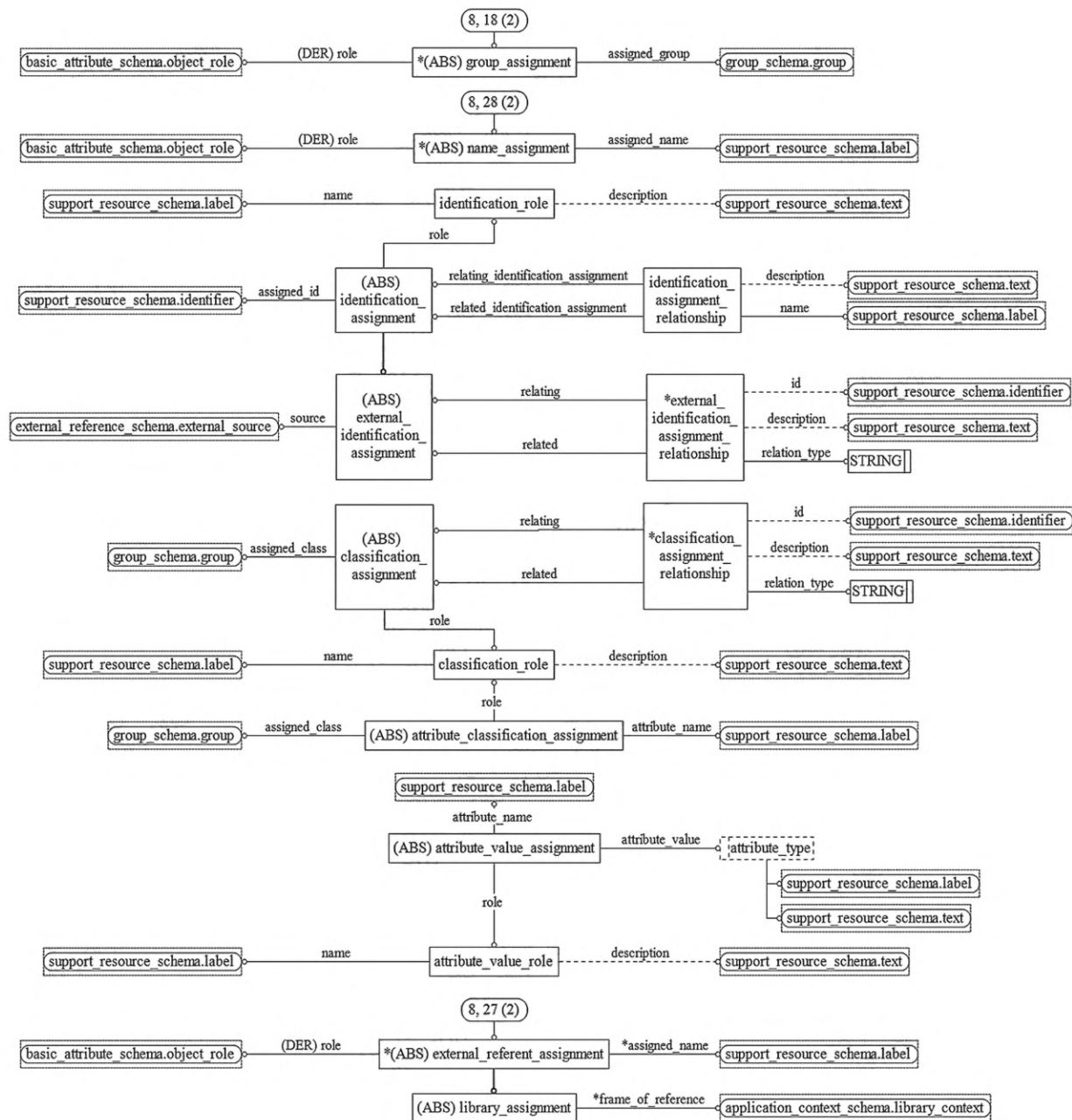
Рисунок D.40 — EXPRESS-G диаграмма схемы management_resources_schema (диаграмма 8 из 9)
