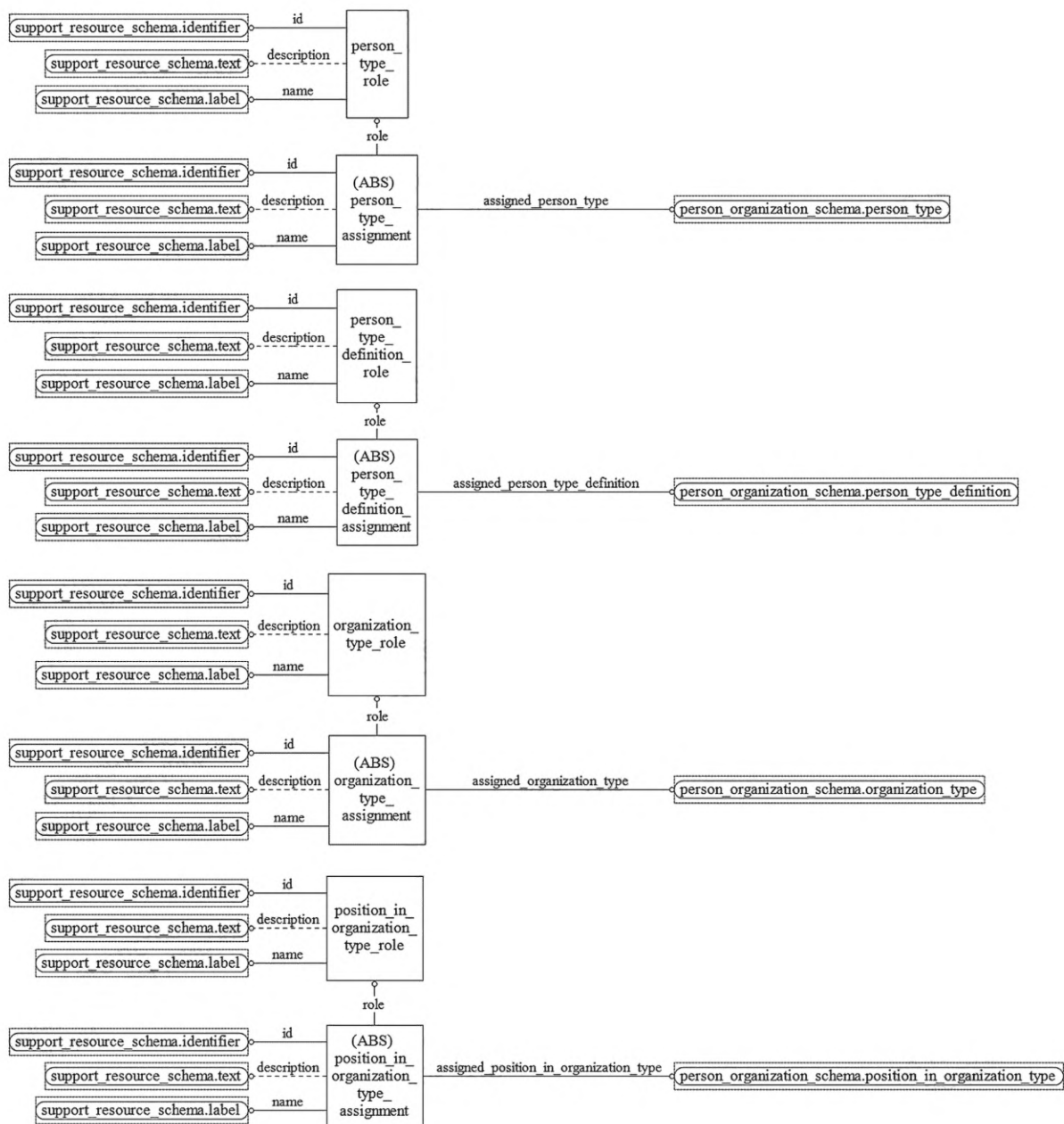
Рисунок D.39 — EXPRESS-G диаграмма схемы management_resources_schema (диаграмма 7 из 9)
