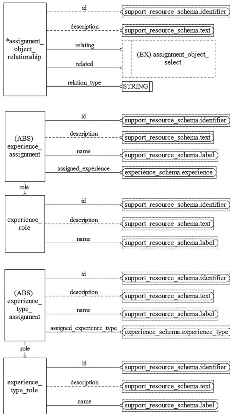
Рисунок D.35 — EXPRESS-G диаграмма схемы management_resources_schema (диаграмма 3 из 9)
