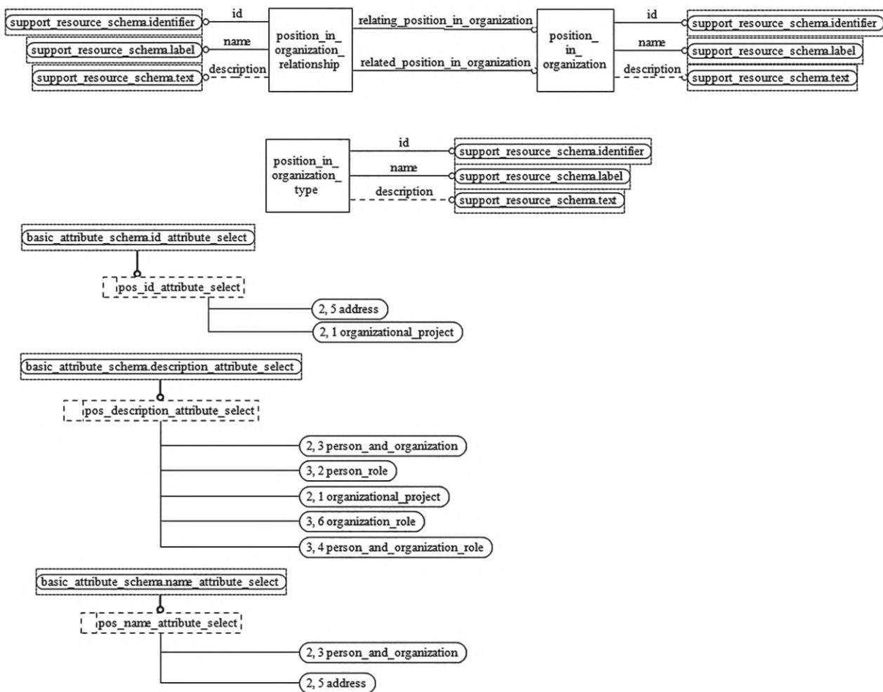
Рисунок D.50 — EXPRESS-G диаграмма схемы person_organization_schema (диаграмма 4 из 4)
