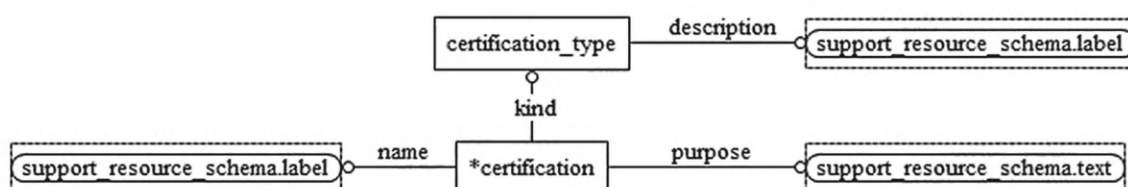
Рисунок D.13 — EXPRESS-G диаграмма схемы certification_schema (диаграмма 2 из 2)
