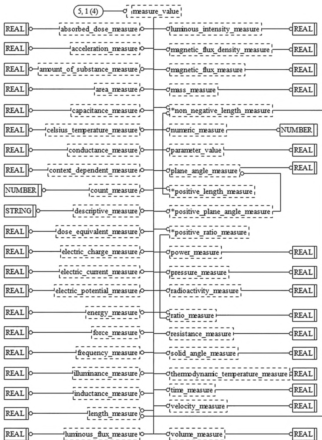
Рисунок D.46 — EXPRESS-G диаграмма схемы measure_schema (диаграмма 5 из 5)
