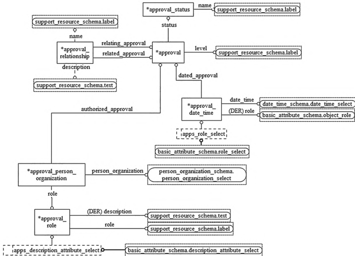
Рисунок D.6 — EXPRESS-G диаграмма схемы approval_schema (диаграмма 2 из 2)
