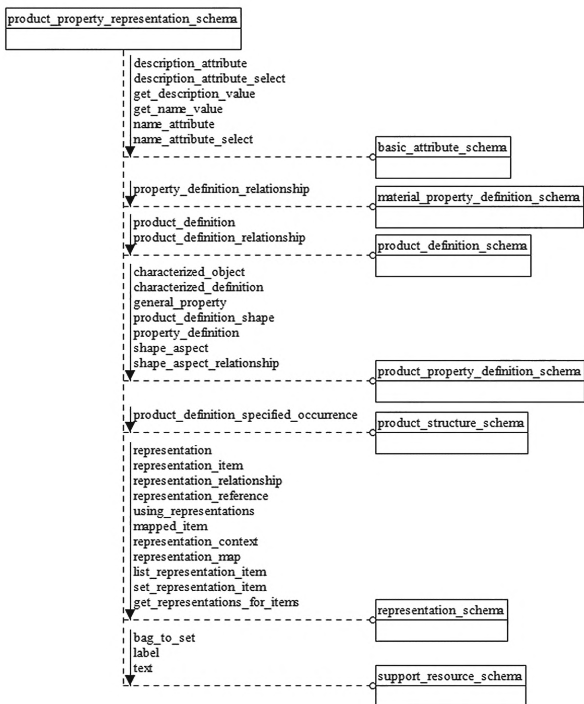
Рисунок D.56 — EXPRESS-G диаграмма схемы product_property_representation_schema (диаграмма 1 из 2)
