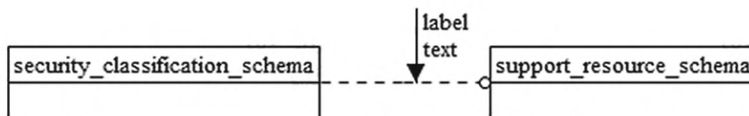
Рисунок D.60 — EXPRESS-G диаграмма схемы security_classification_schema (диаграмма 1 из 2)
