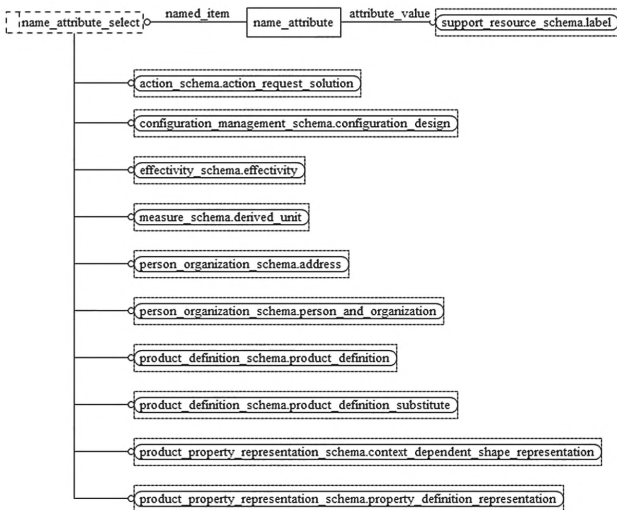
Рисунок D.10 — EXPRESS-G диаграмма схемы basic_attribute_schema (диаграмма 4 из 5)
