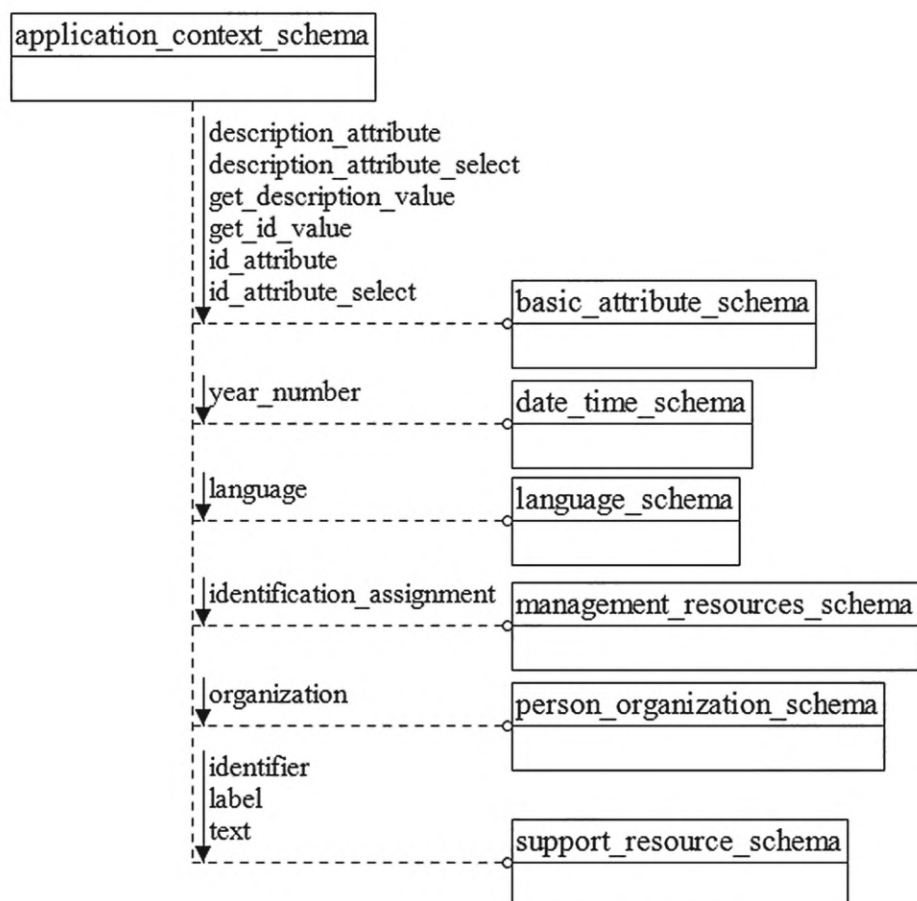
Рисунок D.3 — EXPRESS-G диаграмма схемы application_context_schema (диаграмма 1 из 2)
