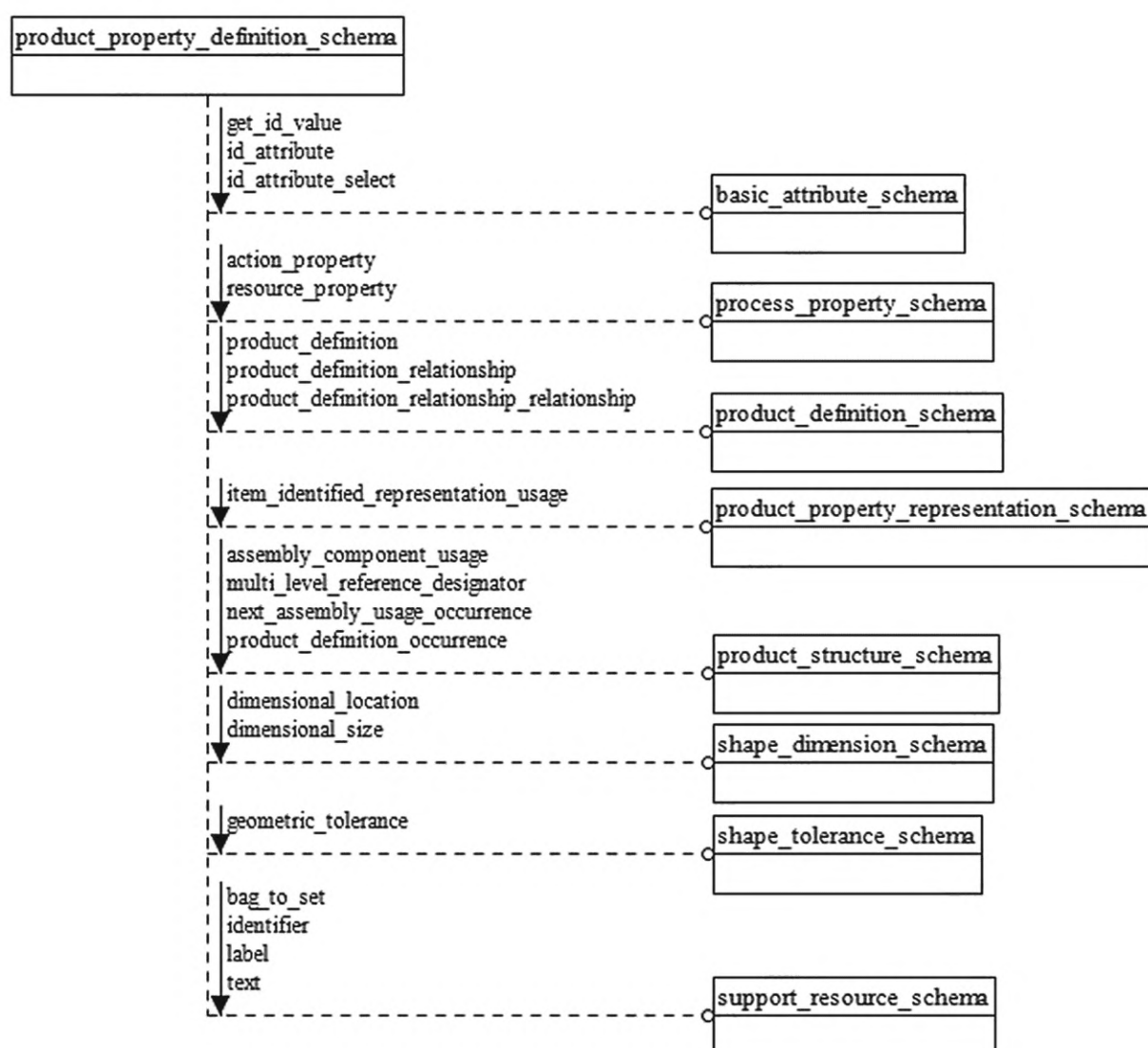
Рисунок D.54 — EXPRESS-G диаграмма схемы product_property_definition_schema (диаграмма 1 из 2)
