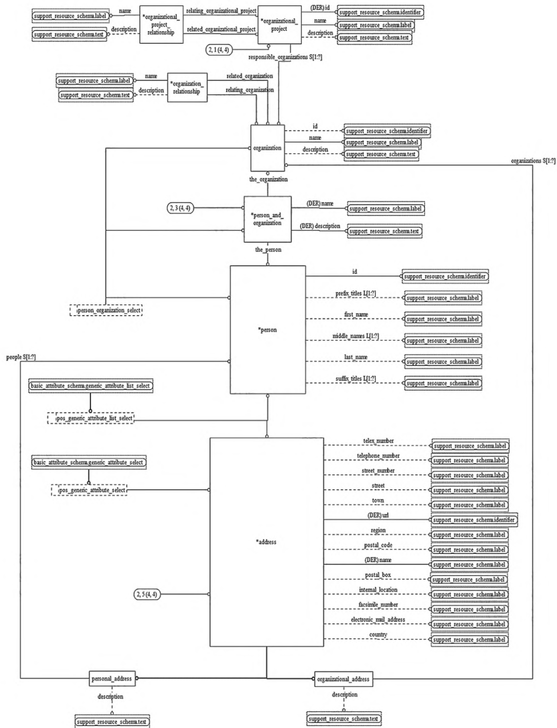
Рисунок D.48 — EXPRESS-G диаграмма схемы person_organization_schema (диаграмма 2 из 4)
