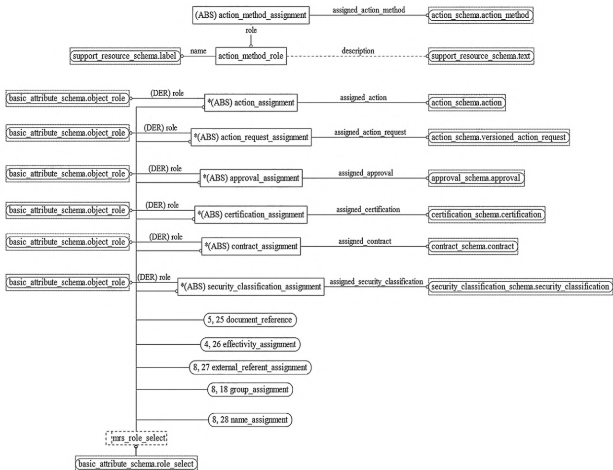
Рисунок D.34 — EXPRESS-G диаграмма схемы management_resources_schema (диаграмма 2 из 9)
