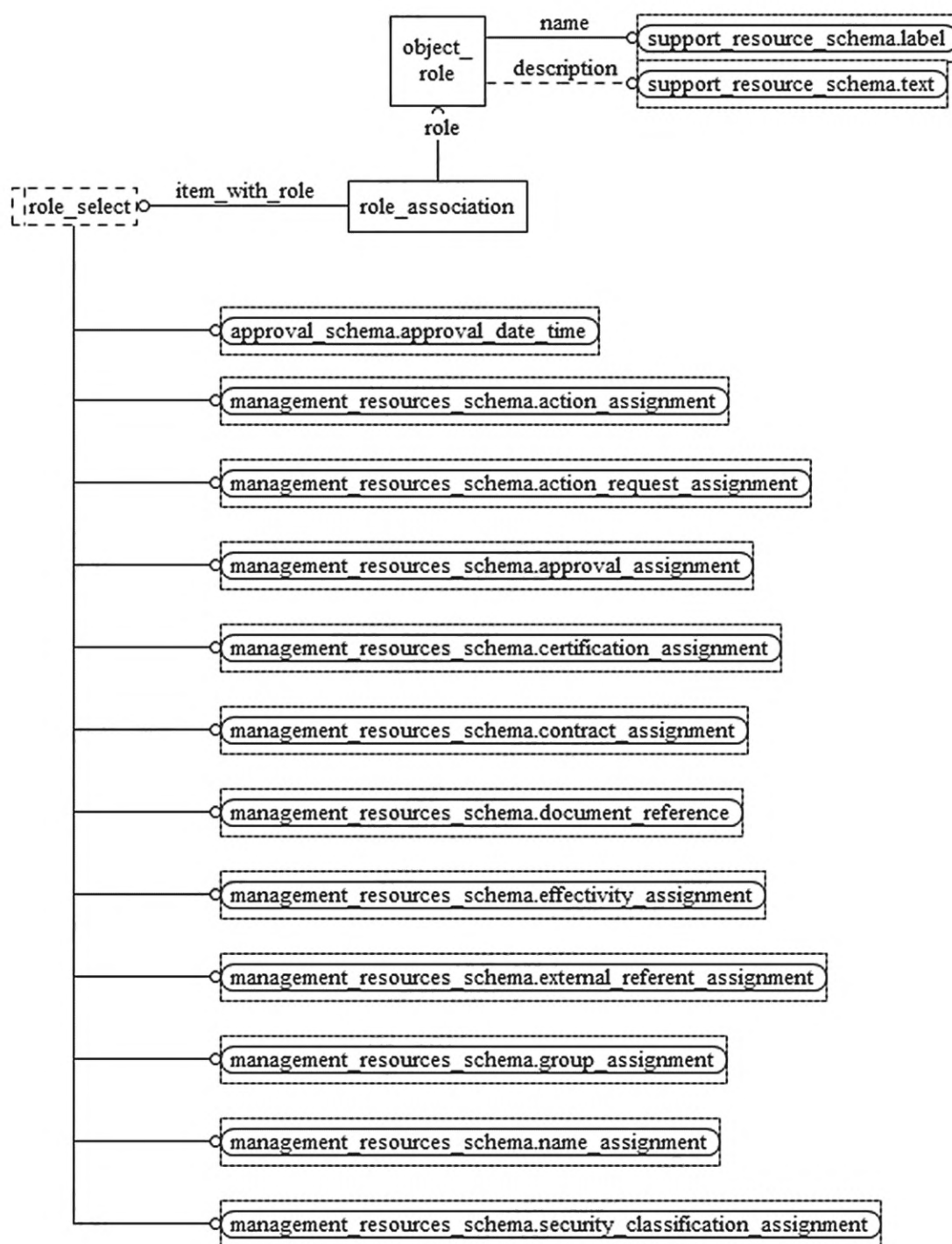
Рисунок D.11 — EXPRESS-G диаграмма схемы basic_attribute_schema (диаграмма 5 из 5)
