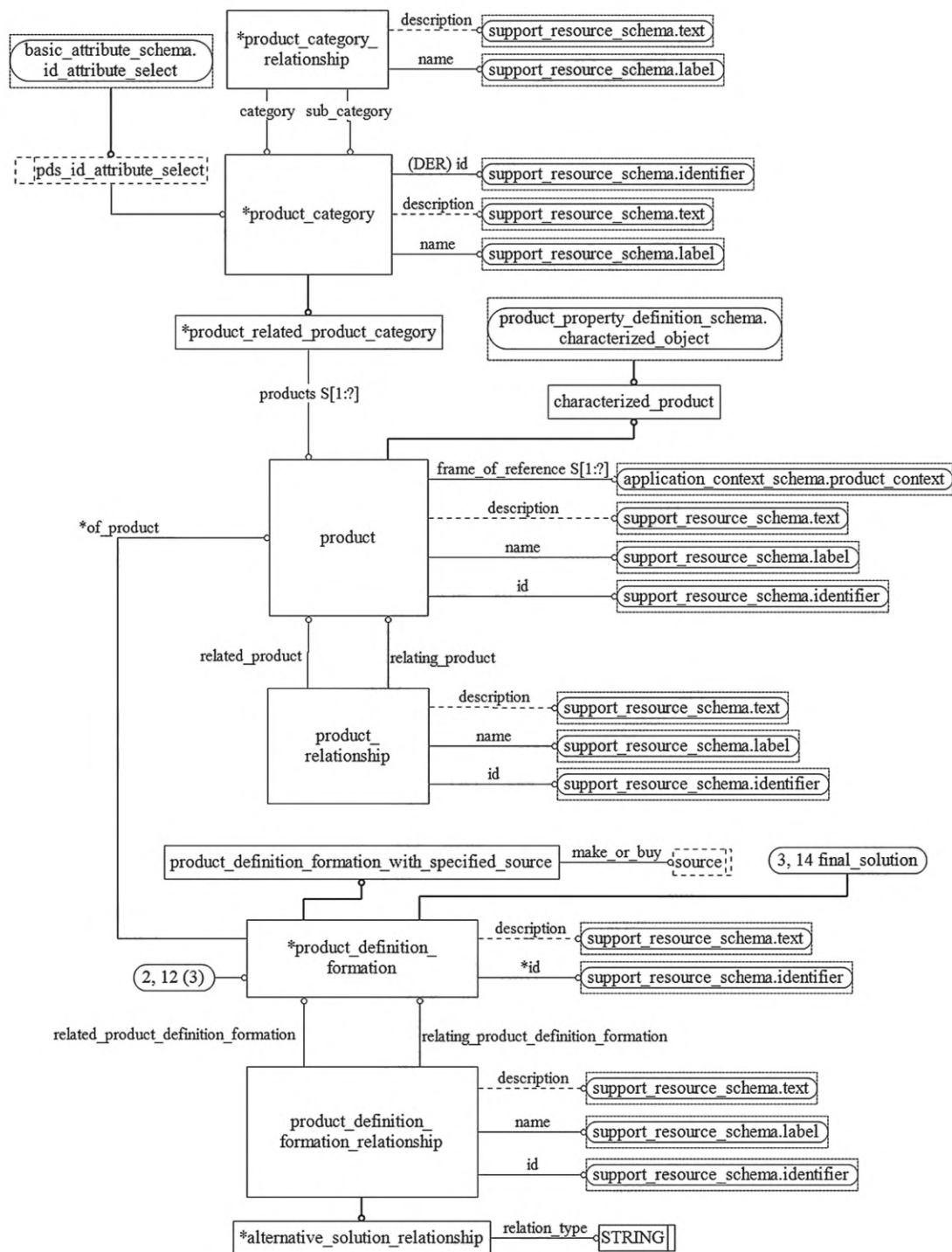
Рисунок D.52 — EXPRESS-G диаграмма схемы product_definition_schema (диаграмма 2 из 3)
