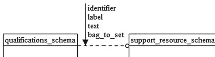
Рисунок D.58 — EXPRESS-G диаграмма схемы qualifications_schema (диаграмма 1 из 2)
