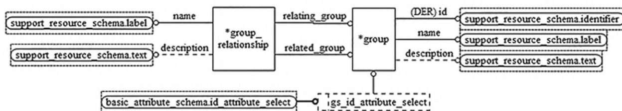
Рисунок D.28 — EXPRESS-G диаграмма схемы group_schema (диаграмма 2 из 2)
