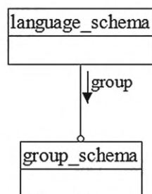
Рисунок D.29 — EXPRESS-G диаграмма схемы language_schema (диаграмма 1 из 2)
