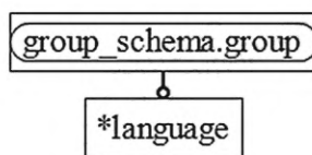
Рисунок D.30 — EXPRESS-G диаграмма схемы languagee_schema (диаграмма 2 из 2)
