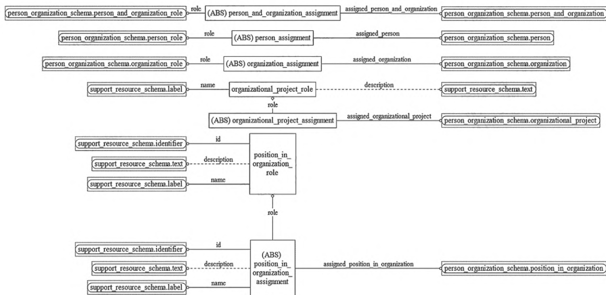
Рисунок D.38 — EXPRESS-G диаграмма схемы management_resources_schema (диаграмма 6 из 9)
