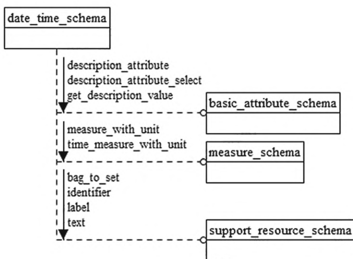
Рисунок D.16 — EXPRESS-G диаграмма схемы date_time_schema (диаграмма 1 из 3)
