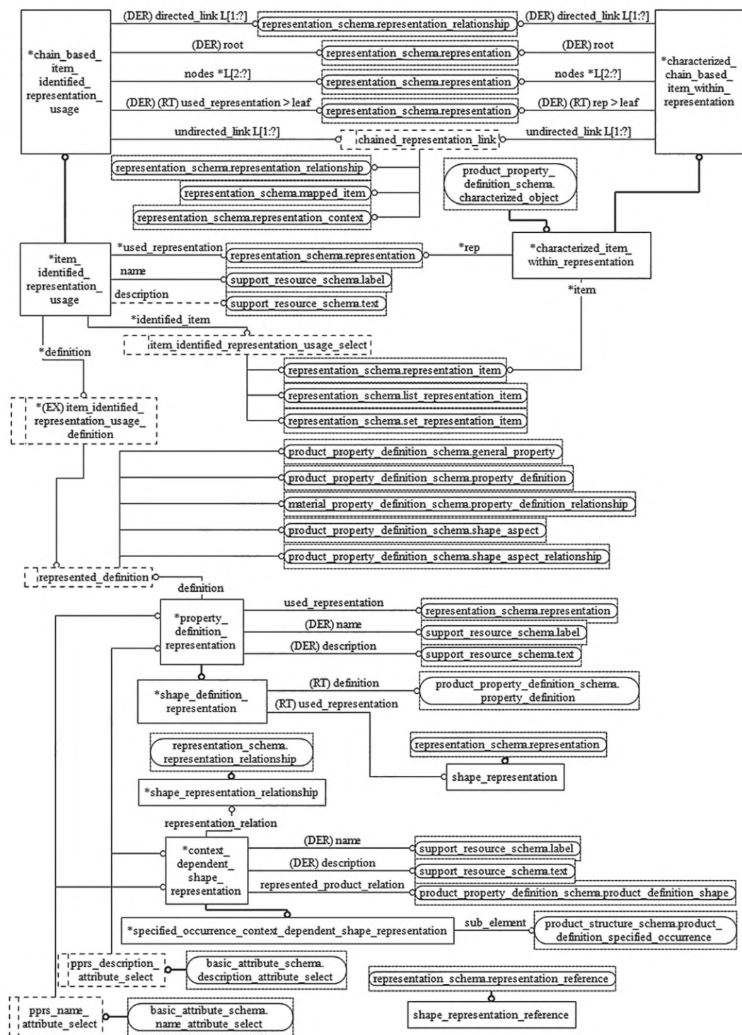
Рисунок D.57 — EXPRESS-G диаграмма схемы product_property_representation_schema (диаграмма 2 из 2)
