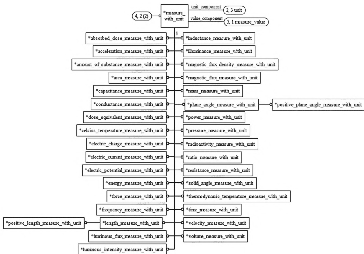
Рисунок D.45 — EXPRESS-G диаграмма схемы measure_schema (диаграмма 4 из 5)
