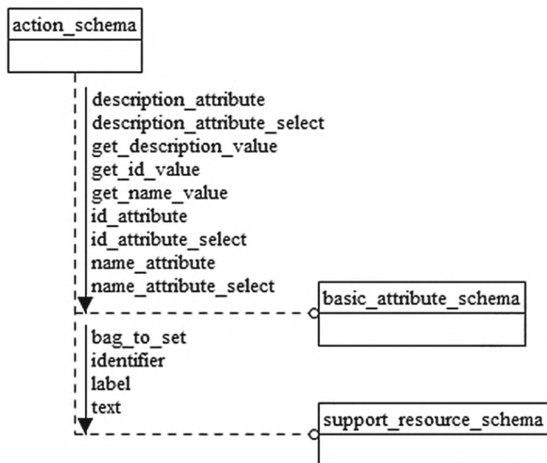
Рисунок D.1 — EXPRESS-G диаграмма схемы action_schema (диаграмма 1 из 2)
