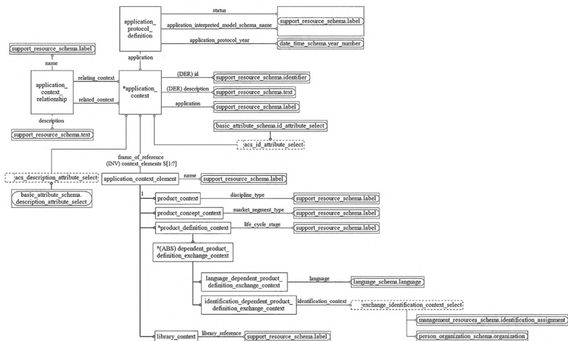
Рисунок D.4 — EXPRESS-G диаграмма схемы application_context_schema (диаграмма 2 из 2)
