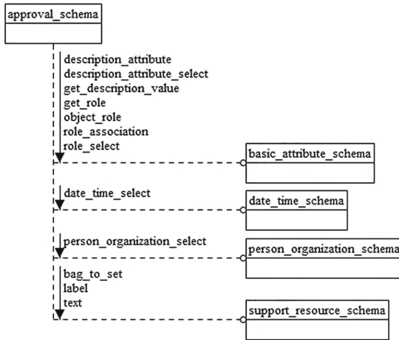
Рисунок D.5 — EXPRESS-G диаграмма схемы approval_schema (диаграмма 1 из 2)
