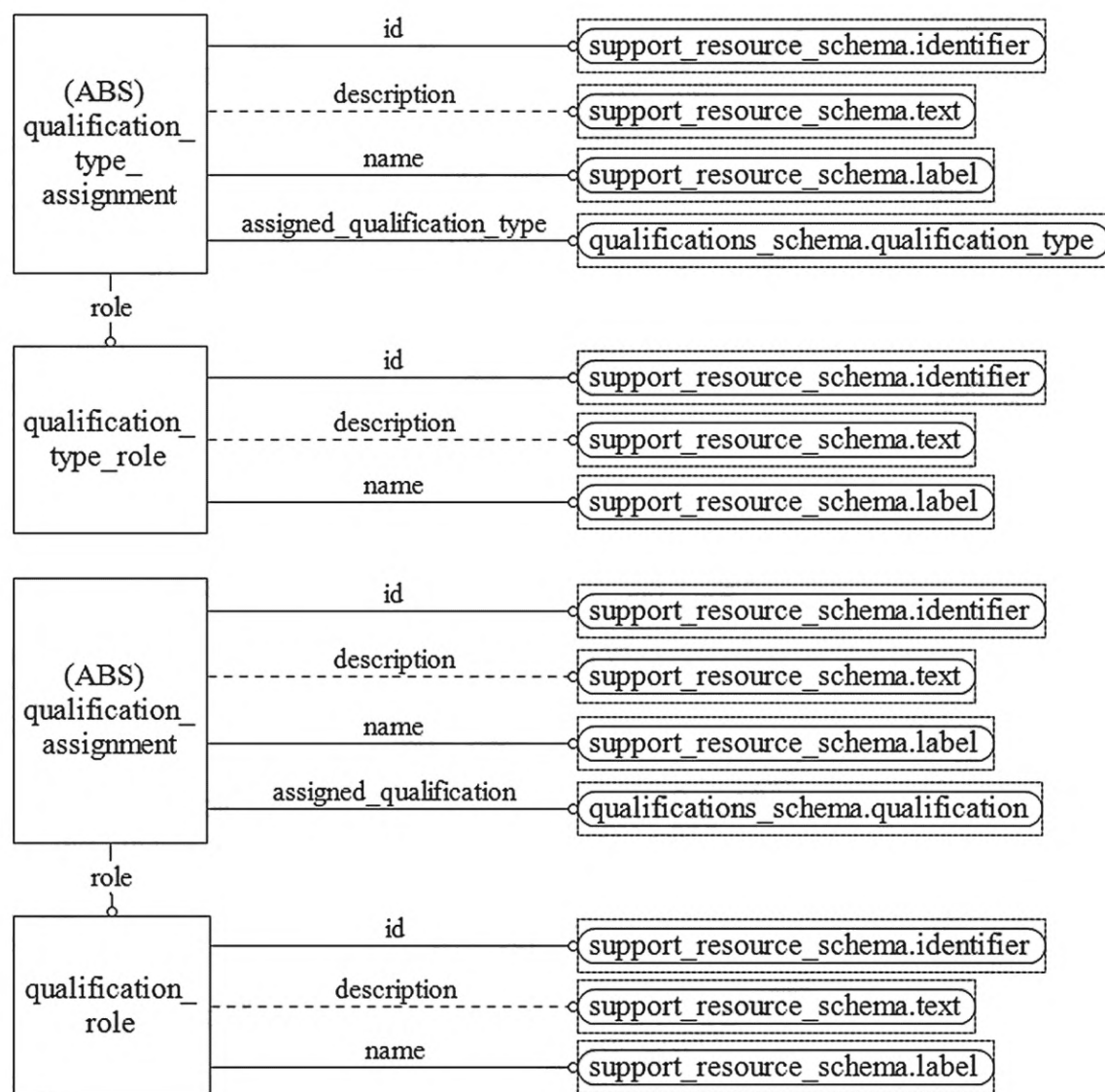
Рисунок D.41 — EXPRESS-G диаграмма схемы management_resources_schema (диаграмма 9 из 9)
