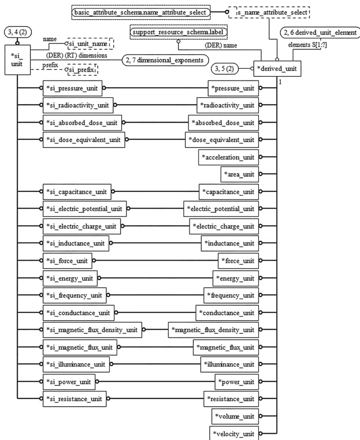
Рисунок D.44 — EXPRESS-G диаграмма схемы measure_schema (диаграмма 3 из 5)
