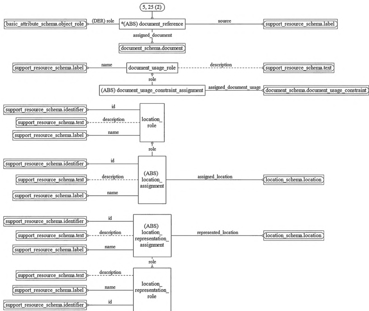
Рисунок D.37 — EXPRESS-G диаграмма схемы management_resources_schema (диаграмма 5 из 9)
