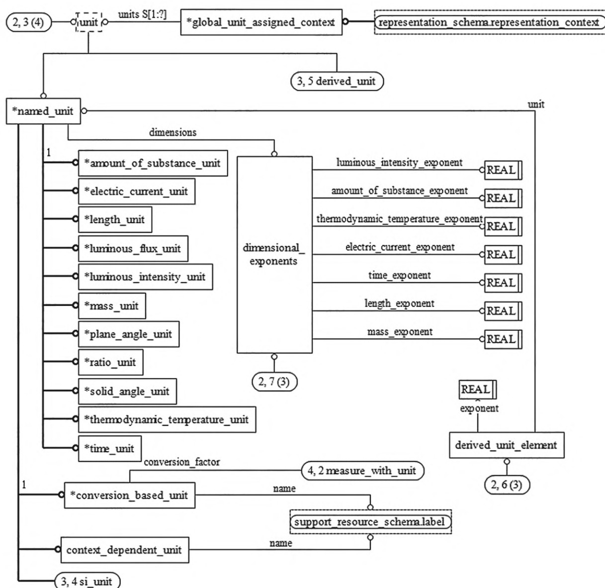
Рисунок D.43 — EXPRESS-G диаграмма схемы measure_schema (диаграмма 2 из 5)
