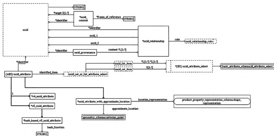
Рисунок D.65 — EXPRESS-G диаграмма схемы uuid_attribute_schema (диаграмма 2 из 2)
