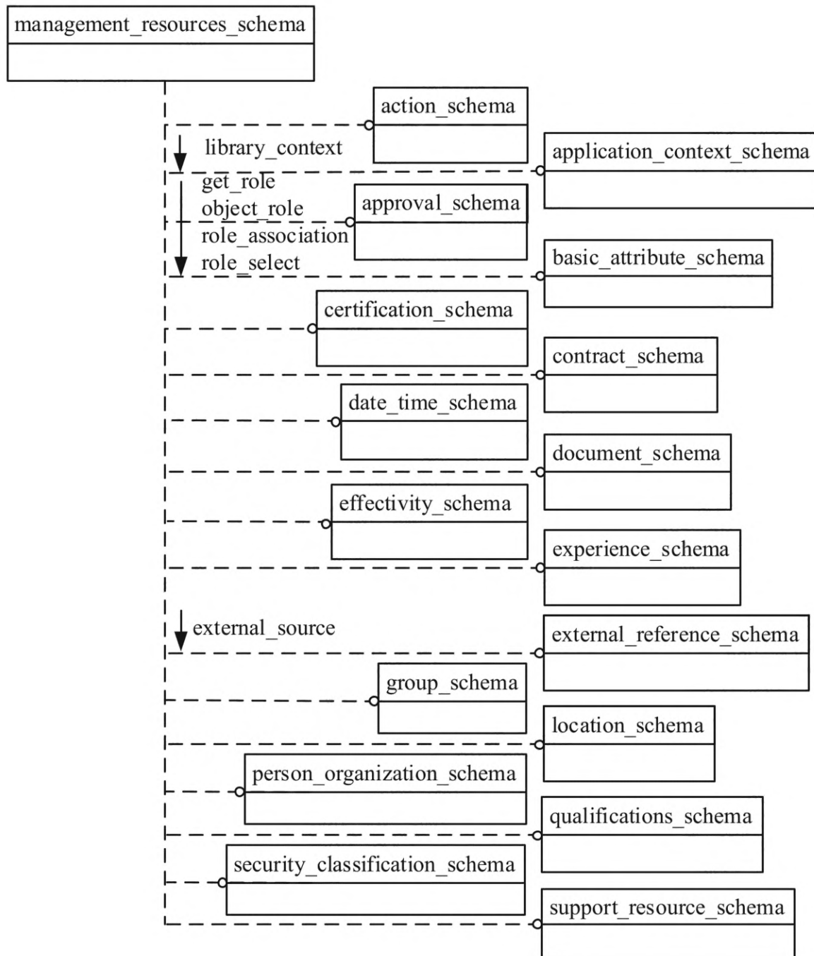
Рисунок D.33 — EXPRESS-G диаграмма схемы management_resources_schema (диаграмма 1 из 9)
