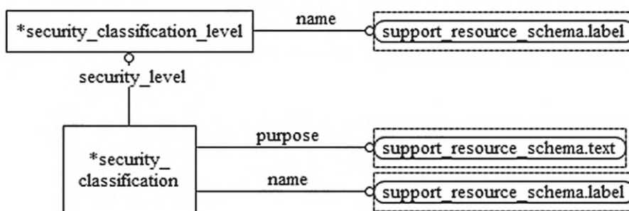
Рисунок D.61 — EXPRESS-G диаграмма схемы security_classification_schema (диаграмма 2 из 2)
