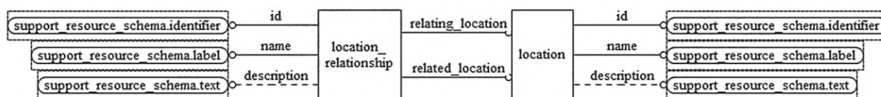
Рисунок D.32 — EXPRESS-G диаграмма схемы location_schema (диаграмма 2 из 2)
