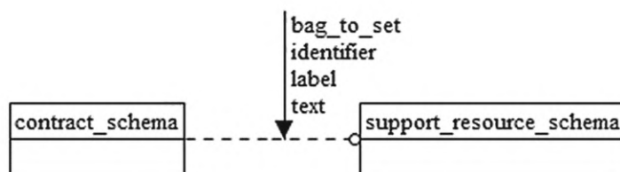
Рисунок D.14 — EXPRESS-G диаграмма схемы contract_schema (диаграмма 1 из 2)
