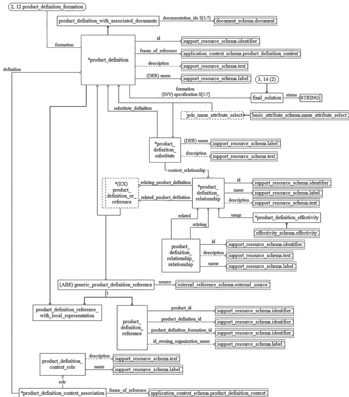
Рисунок D.53 — EXPRESS-G диаграмма схемы product_definition_schema (диаграмма 3 из 3)
