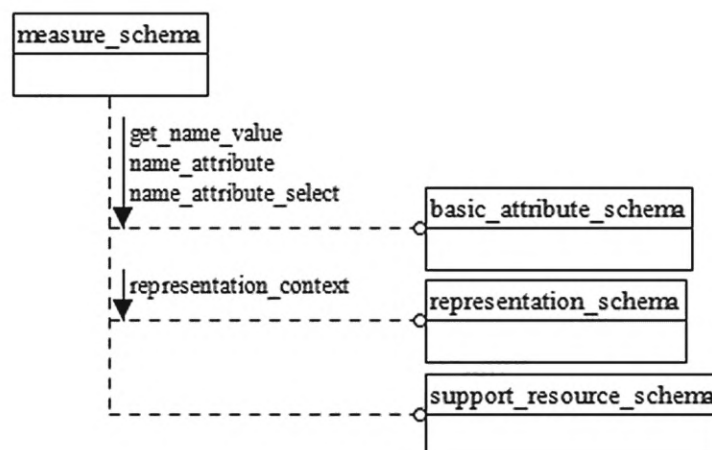
Рисунок D.42 — EXPRESS-G диаграмма схемы measure_schema (диаграмма 1 из 5)
