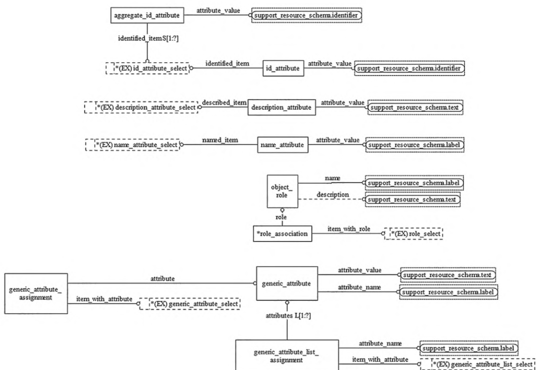
Рисунок D.8 — EXPRESS-G диаграмма схемы basic_attribute_schema (диаграмма 2 из 5)
