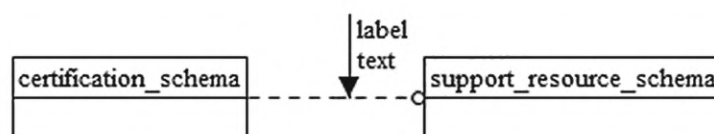
Рисунок D.12 — EXPRESS-G диаграмма схемы certification_schema (диаграмма 1 из 2)
