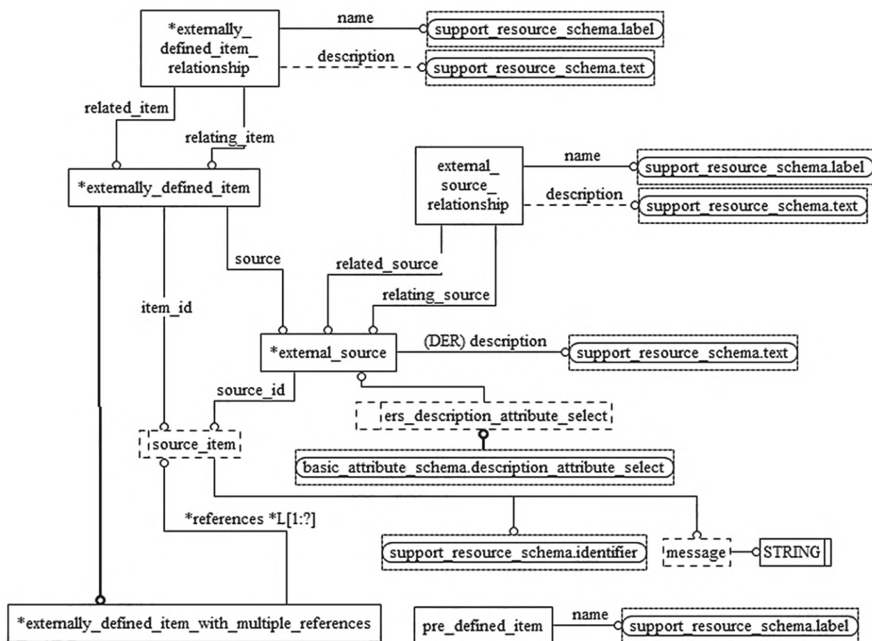
Рисунок D.26 — EXPRESS-G диаграмма схемы external_reference_schema (диаграмма 2 из 2)
