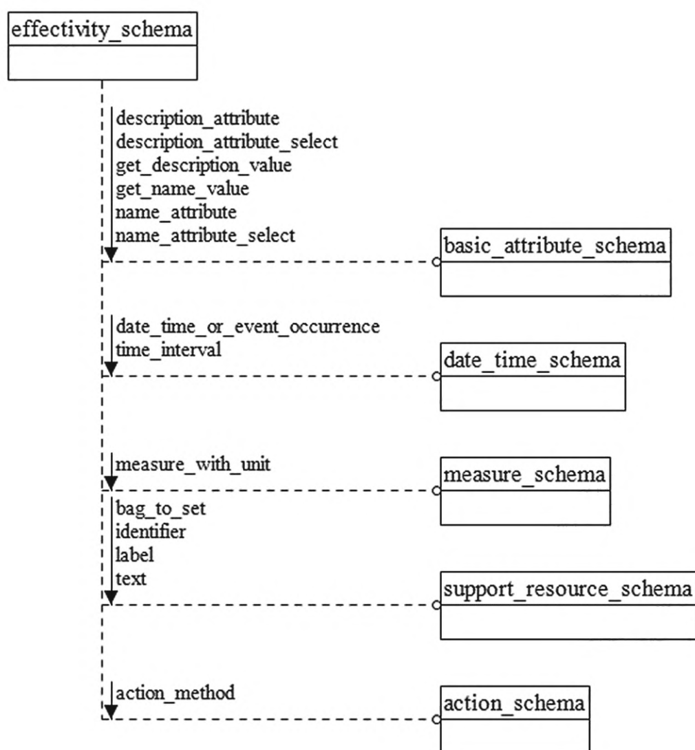
Рисунок D.21 — EXPRESS-G диаграмма схемы effectivity_schema (диаграмма 1 из 2)
