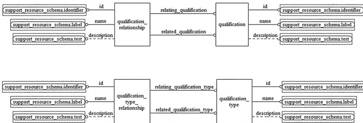
Рисунок D.59 — EXPRESS-G диаграмма схемы qualifications_schema (диаграмма 2 из 2)
