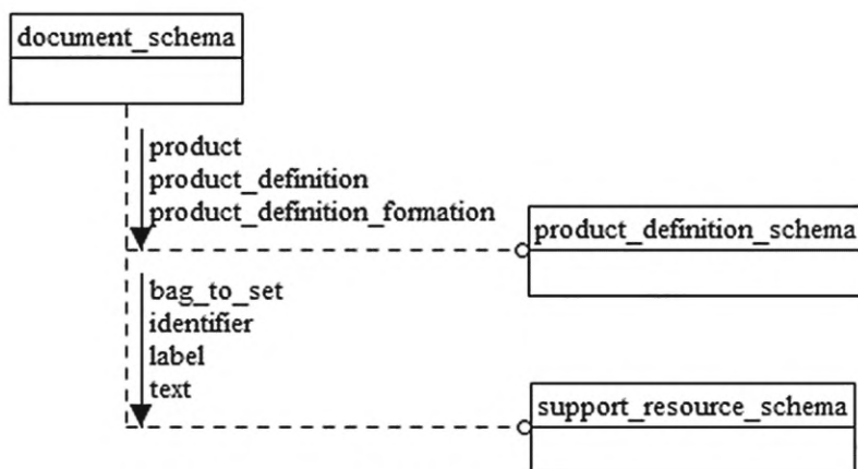
Рисунок D.19 — EXPRESS-G диаграмма схемы document_schema (диаграмма 1 из 2)
