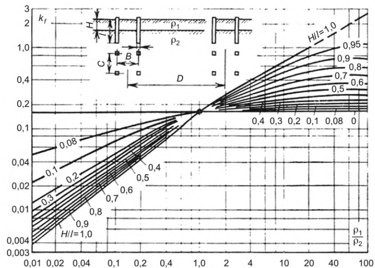
Рисунок Б.11 — Коэффициент формы k_f в зависимости от \rho_1/\rho_2 и H/l для восьмисвайного фундамента portalной опоры при a/l = 0,05 , B/C = 1,0 , B/l = 1,0 , D/l = 3,0
