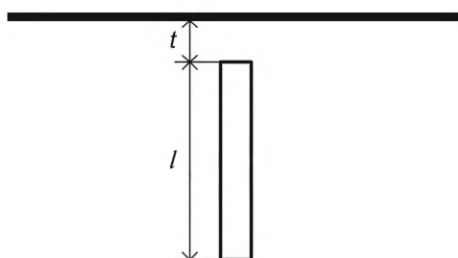
Рисунок Б.5 — Вертикальный заземлитель
