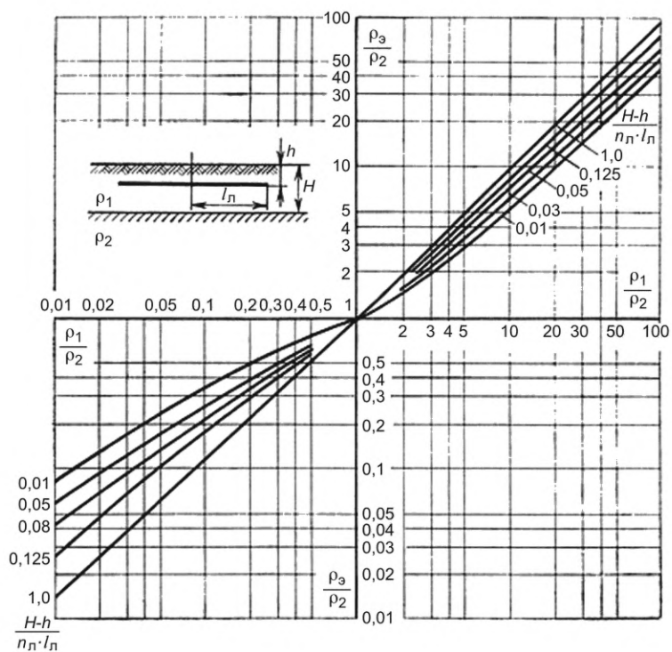
Рисунок Б.2 — Относительное эквивалентное удельное сопротивление грунта для расчета n -лучевых заземлителей
