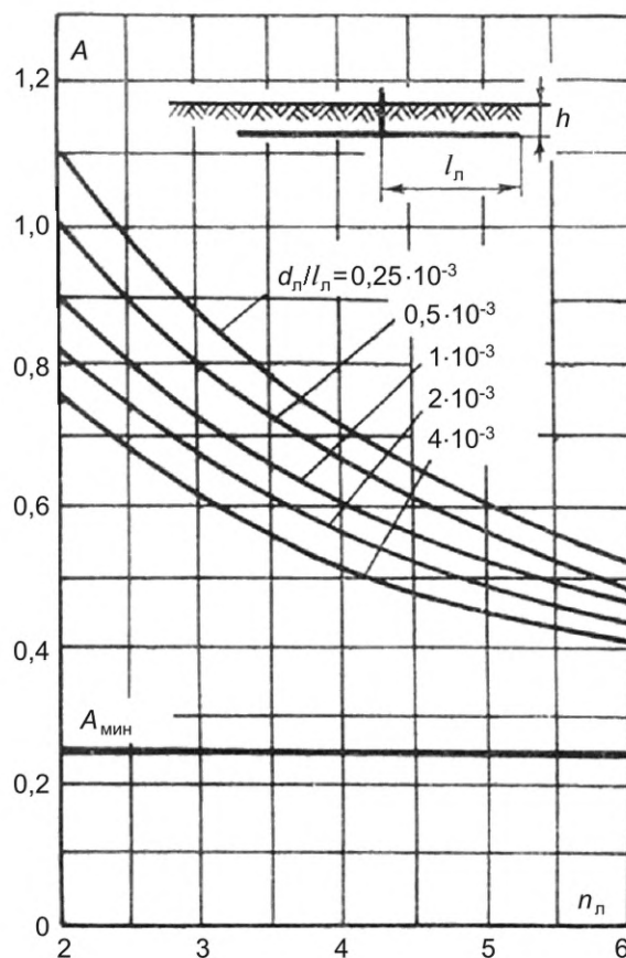
Рисунок Б.7 — Коэффициент подобия A для лучевых заземлителей в зависимости от числа лучей n_n и отношения диаметра d_n к длине электрода l_n
