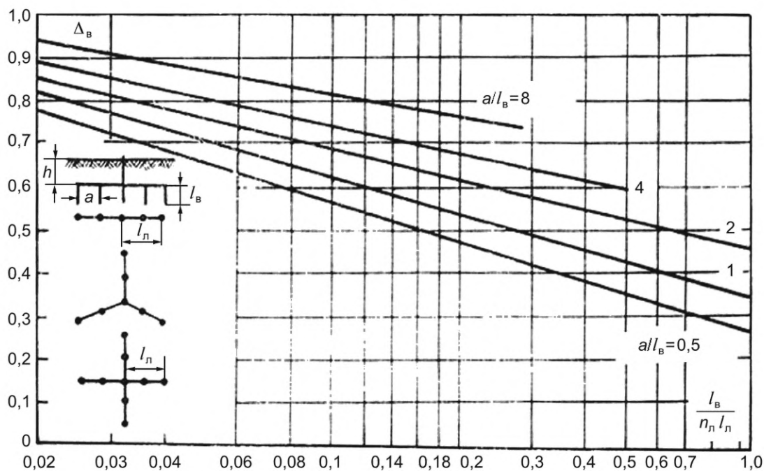
Рисунок Б.8 — Зависимость коэффициента \Delta_B от добавления вертикальных электродов
