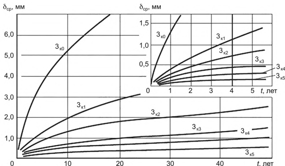
Рисунок 1 — Зависимость глубины коррозии стальных заземлителей \delta_{ср} от времени для различных коррозионных зон
