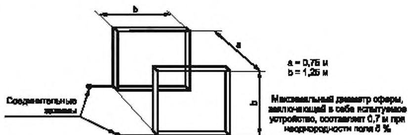
Рисунок A.1 — Конструкция катушки Гельмгольца для однородных полей
