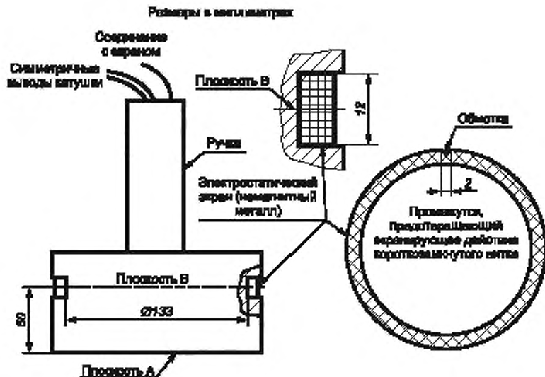
Рисунок A.2 — Конструкция излучающей рамки для неоднородных полей
