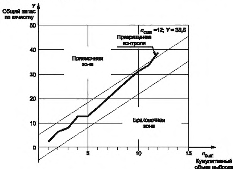
Рисунок 8 — Приемочная карта для последовательного плана выборочного контроля при одностороннем допуске (пример 3.5.1.3)
