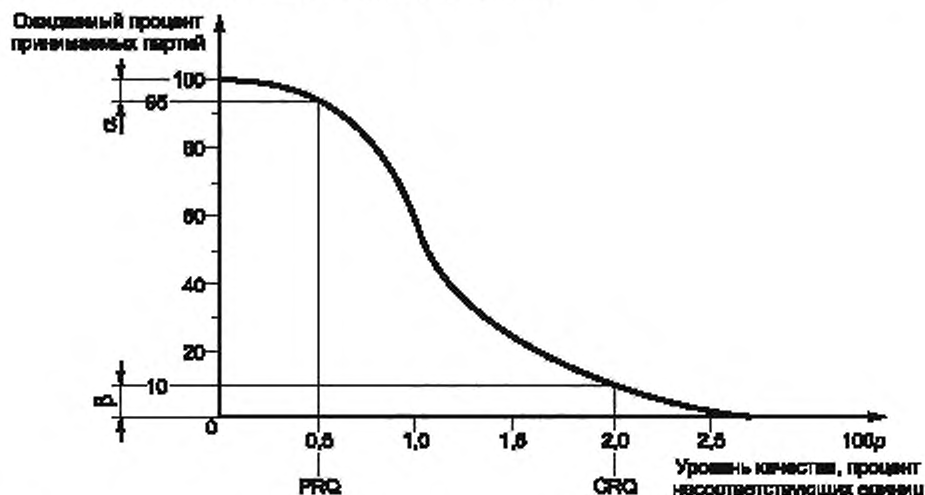
Рисунок 1 — Оперативная характеристика плана выборочного контроля с параметрами: риск поставщика \alpha = 0,05 , риск потребителя \beta = 0,10
