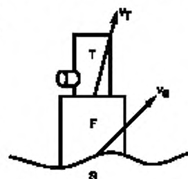
Рисунок 1 — Схематическое изображение установки акселерометра
