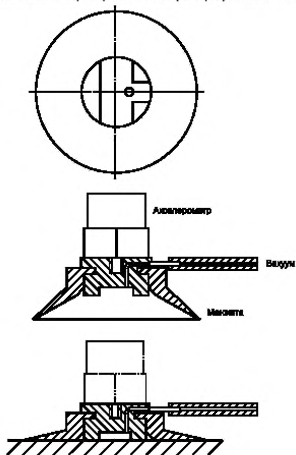
Рисунок 11 — Вакуумное крепление
