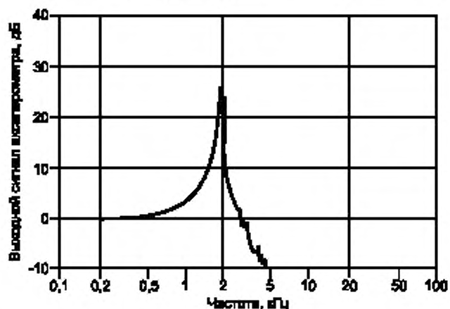
Рисунок 8 — Типичная частотная характеристика акселерометра с щупом
