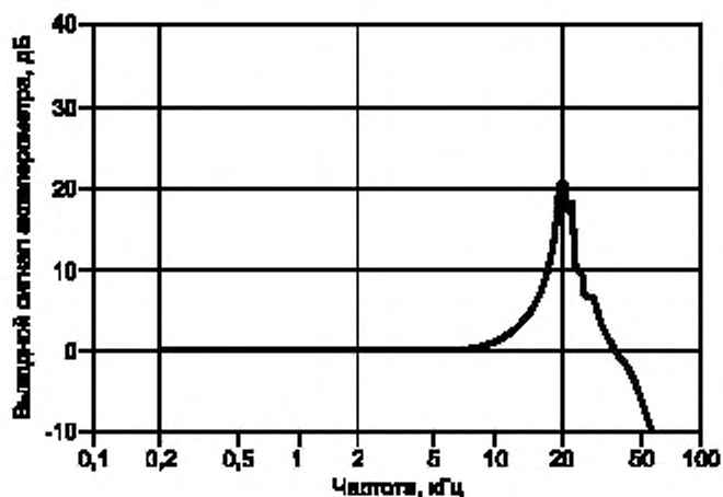
Рисунок 9 — Типичная частотная характеристика акселерометра на магните
