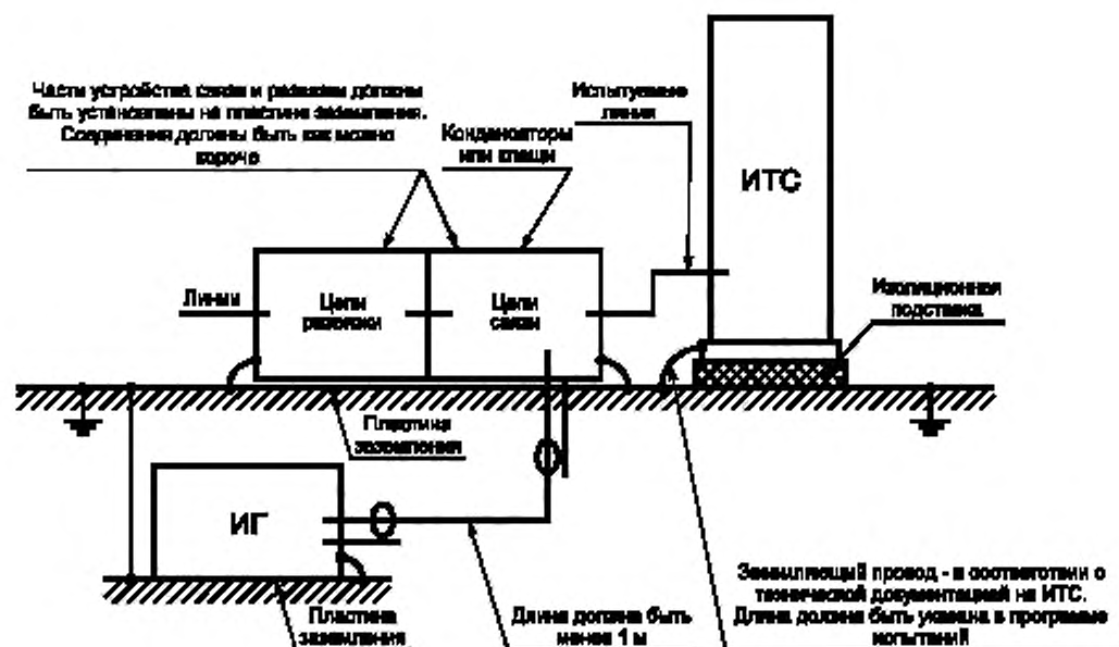
Рисунок 6 — Схема испытаний на устойчивость к НИП
