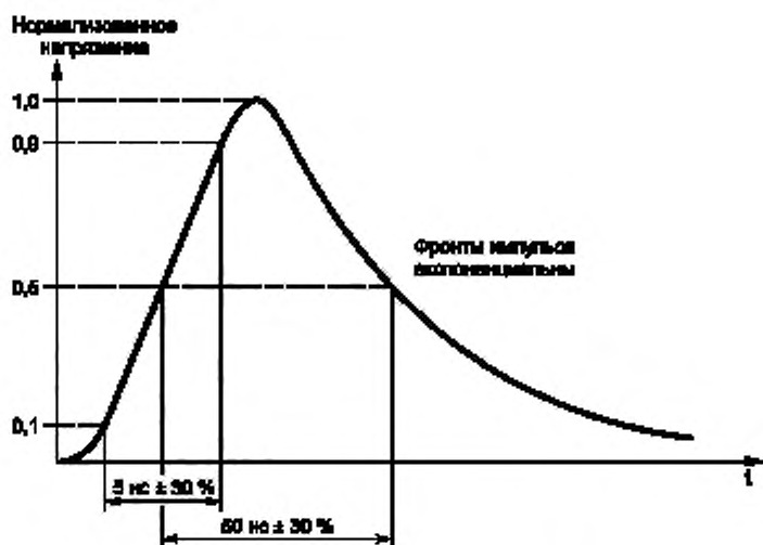
Рисунок 3 — Типовая форма импульса напряжения на нагрузке 50 Ом
