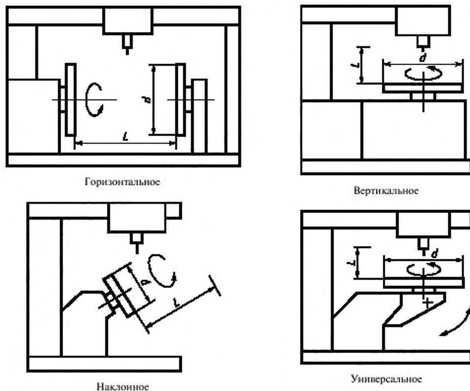
Рисунок 1 – Исполнения оборудования в зависимости от расположения оси вращения изделия
