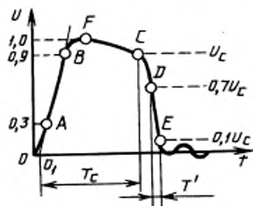
Рисунок 9 — Грозовой импульс, срезанный на спаде импульса
