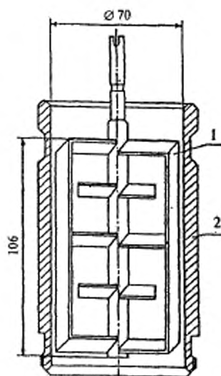
Рисунок 4 — Схема измерительного узла консистометра
