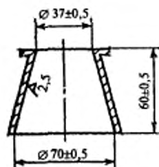
Рисунок 2 — Форма-конус
