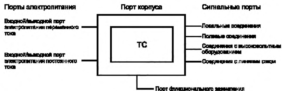
Рисунок 1 — Порты ТС
