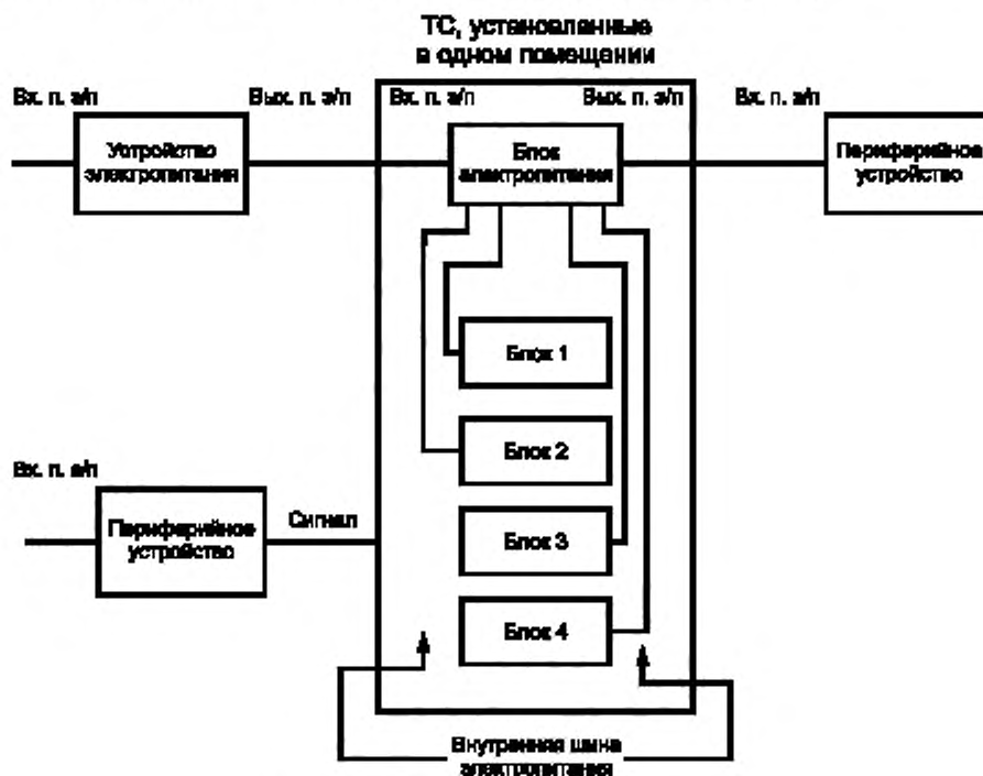
Рисунок 2 — Примеры портов электропитания
