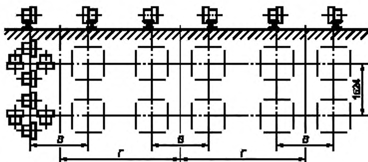
Рисунок Г.4 — Трансформаторы массой от 300 до 700 т
