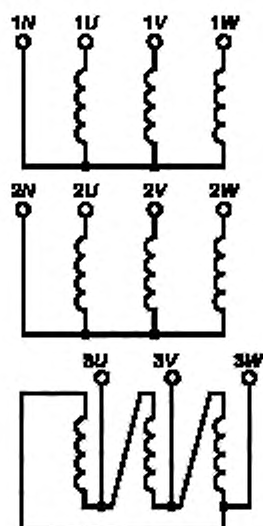
Рисунок Ж.5 — Маркировка трехфазного трехобмоточного трансформатора ( Y_n/Y_n/D-0-5 )
