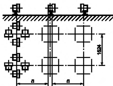
Рисунок Г.2 — Трансформаторы массой от 200 до 255 т
