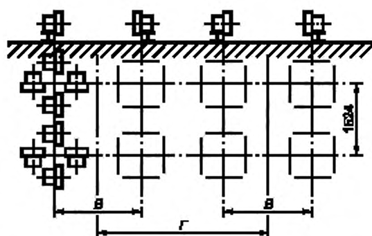
Рисунок Г.3 — Трансформаторы массой от 255 до 300 т
