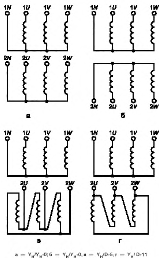
Рисунок Ж.4 — Маркировка трехфазных двухобмоточных трансформаторов
