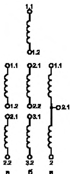
а — трансформатор с двумя обмотками без ответвлений; б — трансформатор с тремя обмотками без ответвлений; в — автотрансформатор без ответвлений
