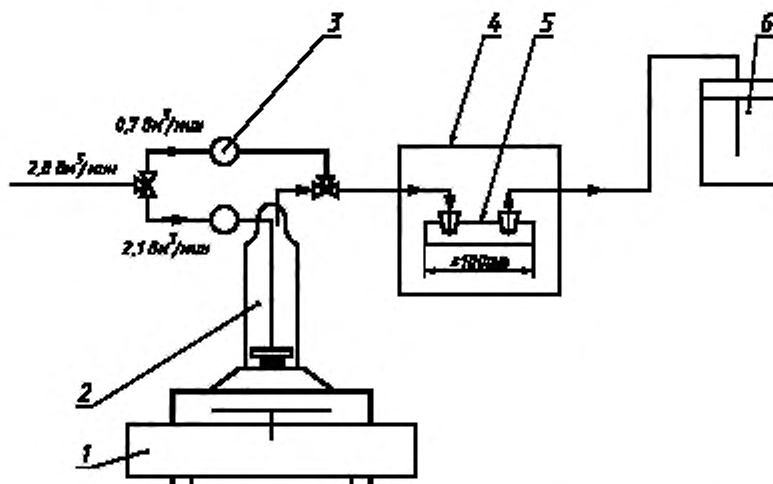
1 — магнитная мешалка; 2 — реакционный сосуд; 3 — газовый фильтр; 4 — атомно-абсорбционный спектрофотометр; 5 — измерительная клетка; 6 — устройство для поглощения паров ртути
