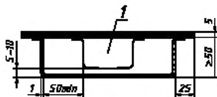
Рисунок 7 — Испытательный кожух для тепловых испытаний ПРА
