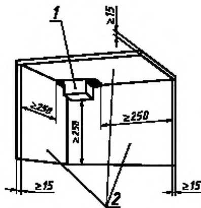
Рисунок 6 — Испытательный угол для тепловых испытаний ПРА
