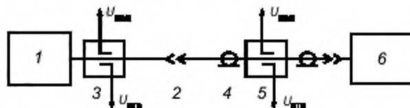
1 — передатчик; 2 — вход антенно-фидерного тракта (выход передатчика); 3 — рефлектометр на выходе передатчика; 4 — фидер антенны; 5 — рефлектометр, установленный в фидерном тракте антенны; 6 — антенна
