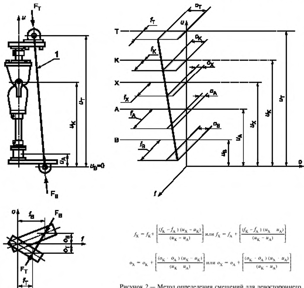
Рисунок 2 — Метод определения смещений для левостороннего образца
