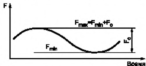
Рисунок 3 — Параметры нагружения при циклических испытаниях
