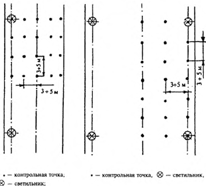
Рисунок А4 — Расположение контрольных точек при измерении средней освещенности улиц при одностороннем однорядном расположении светильников
