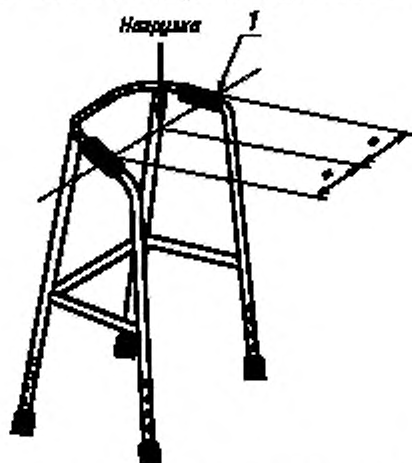
1 — задняя контрольная точка рукоятки
