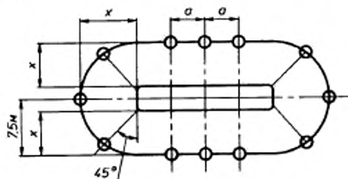
Рисунок А.1 — Положения измерительных точек по контуру транспортного средства на стоянке
