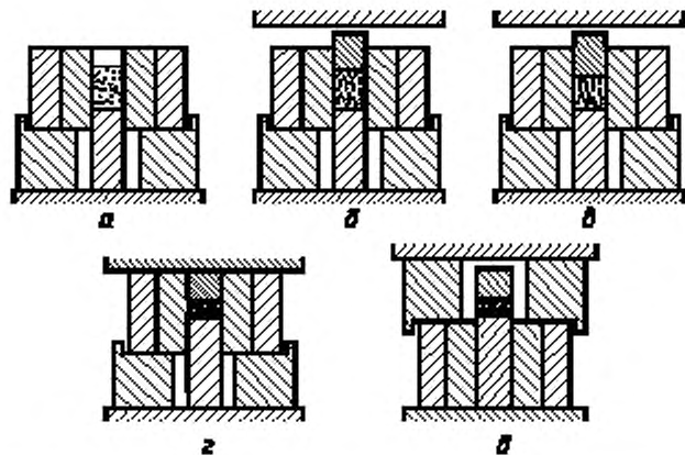
а — закладка порошка в пресс-форму б — установка верхнего пуансона; в — предварительное прессование г — замена опоры и окончательное прессование д — вытягивание
