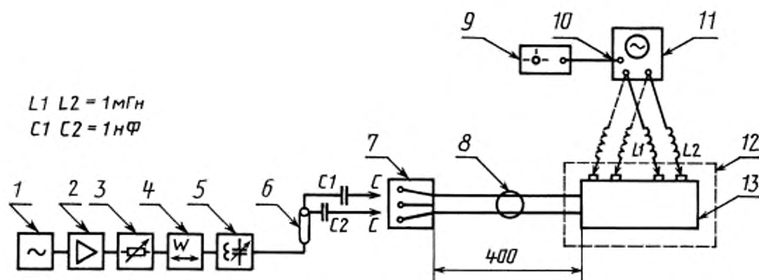
1 — высокочастотный генератор; 2 — высокочастотный усилитель; 3 — высокочастотный аттенуатор; 4 — направленный высокочастотный ваттметр; 5 — согласующее устройство; 6 — коаксиальный кабель 50 Ом; 7 — устройство дистанционного управления; 8 — кабель дистанционного управления; 9 — низкочастотный генератор; 10 — внешний запуск; 11 — осциллограф с полосой от постоянного тока до значения, не превышающего 10 МГц; 12 — металлическая пластина; 13 — испытуемый СТИМУЛЯТОР
