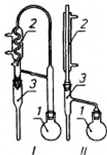
Рисунок 1 — Установка для прямого объемного метода определения влаги
