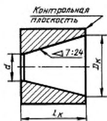
Рисунок 1 — Конусный калибр-штулка
