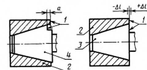
1 — контрольные плоскости; 2 — калибр-втулка, 3 — калибр-пробка контрольный, 4 — калибр-пробка
