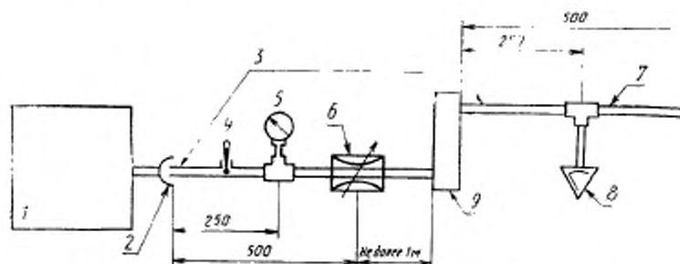
Рисунок № 1 — Испытательное устройство
