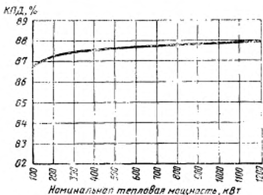
Рисунок 1 — График зависимости КПД рекуперативных воздухогревателей от номинальной тепловой мощности
