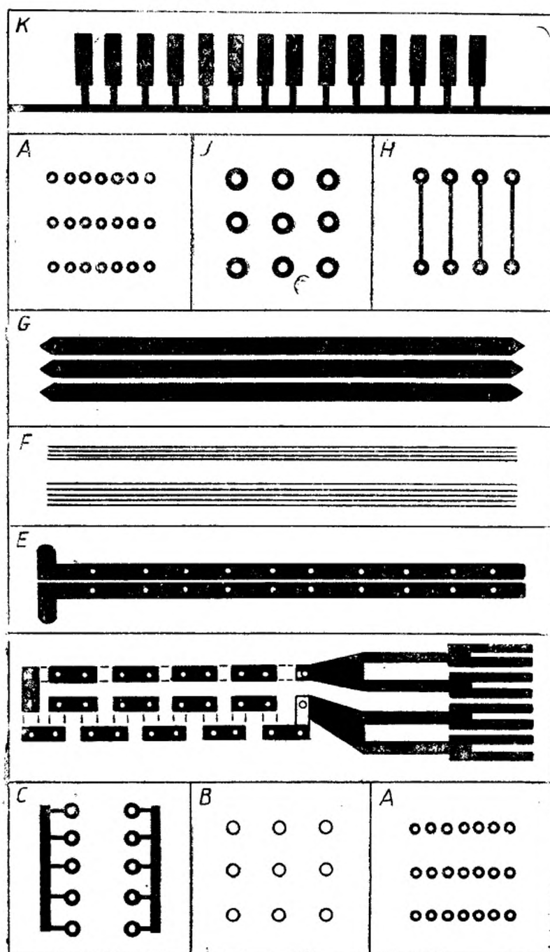
Рисунок 16 — Составной рисунок для испытаний (оборотная сторона)
