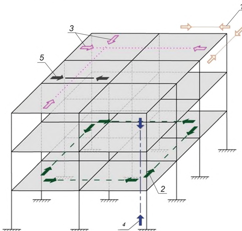
1 — связи по угловым колоннам; 2 — контурные связи; 3 — внутренние связи; 4 — вертикальные связи; 5 — горизонтальные связи по внешним колоннам или стенам
