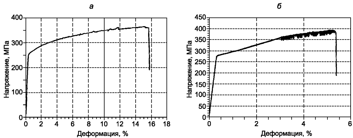
а — алюминиевый деформируемый сплав марки 1915т по ГОСТ 4784; б — алюминиево-магниевый сплав марки 15654 по ГОСТ 4784
