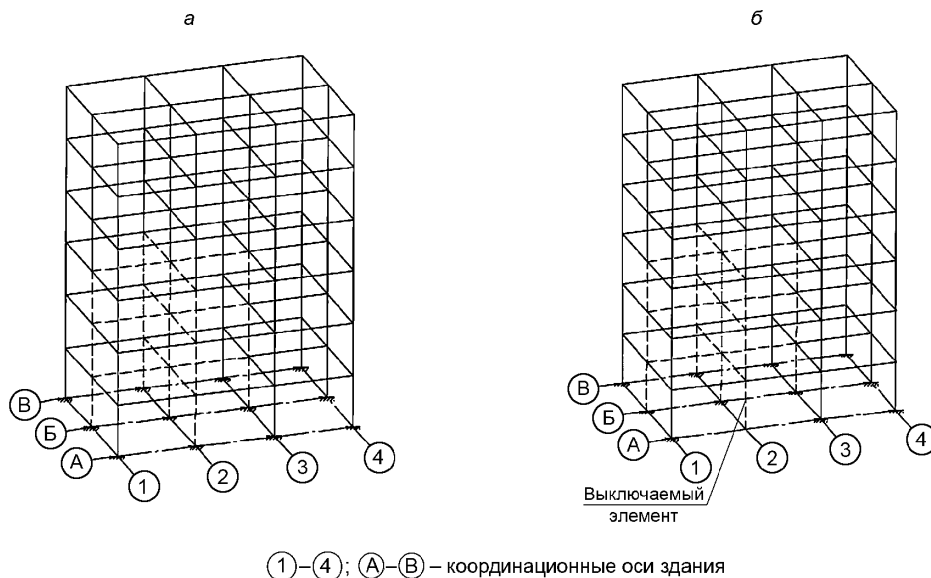
Рисунок 8.1— Первичная (а) и вторичная (б) расчетные схемы здания
