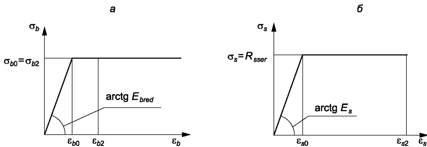
Рисунок К.1 — Диаграммы для определения предельных деформаций бетона (а) и арматуры (б)
