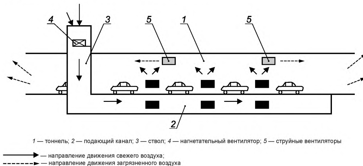
Рисунок 8.6 — Продольно-поперечная схема вентиляции с использованием струйных вентиляторов
