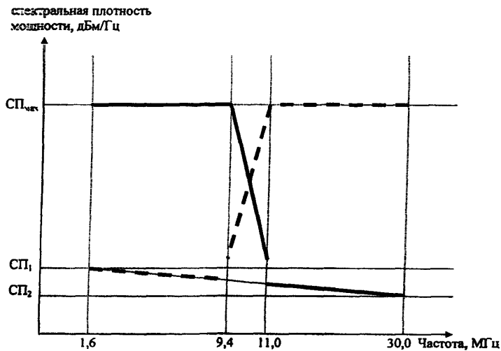
Рис. 6.20. Спектральная плотность мощности выходного сигнала
