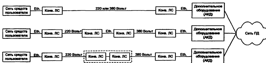
Рис. 6.18. Варианты применения технологии PLT
