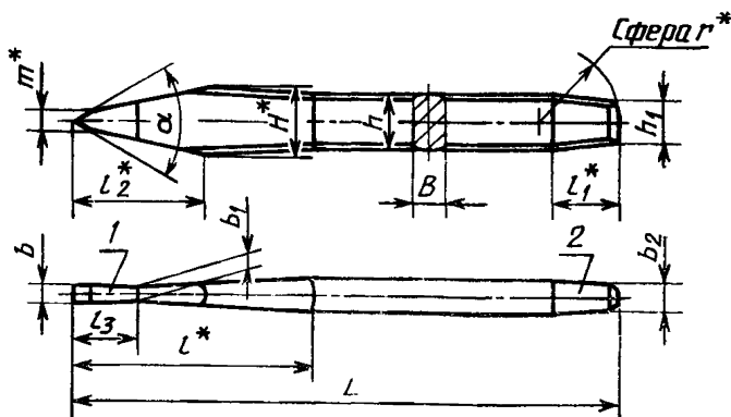
1 — рабочая часть; 2 — ударная часть
