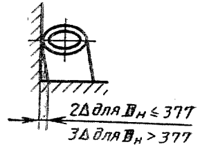
Отвод 45°
