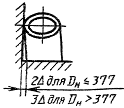
Отвод 60°
