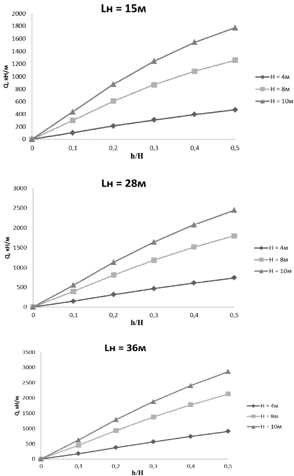
Рисунок 7а - Расчетные графики гидростатического всплытия насыпи с заложением откоса 1:1,5 при коэффициенте запаса 1,1, при трех параметрах ширины дороги
