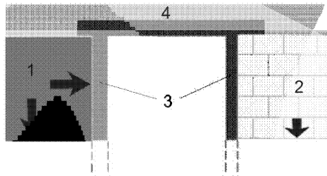
Рисунок 9 - Схема распределения давлений от грунтовой засыпки и засыпки из ППБ. 1 – обратная засыпка грунтом, 2 – укрепление мостового устоя ППБ, 3 – опоры моста, 4 – система дорожной одежды. Стрелками показано распределение давления от грунта обратной засыпки и от ППБ на грунтовое основание и на мостовой устой
