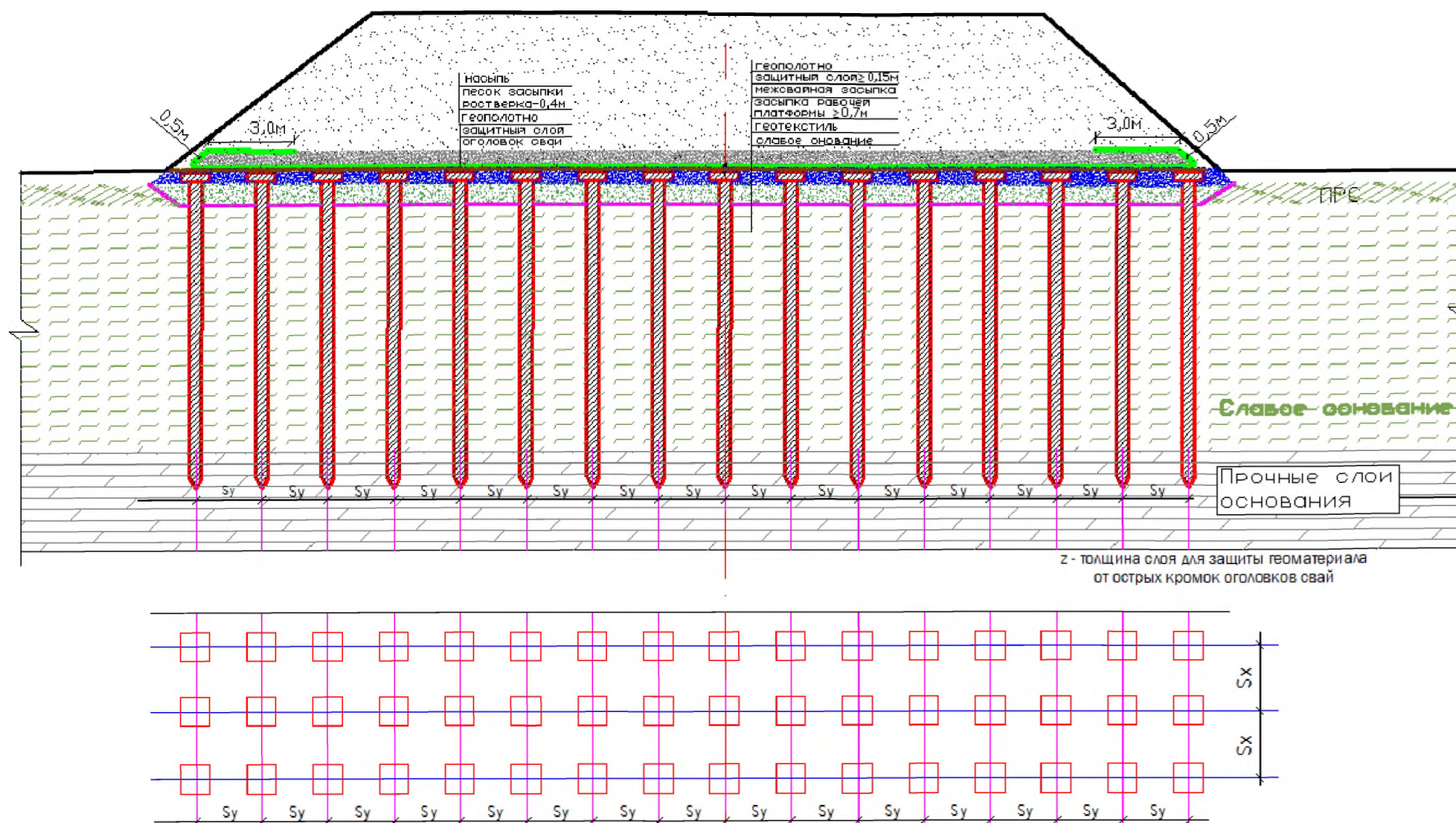
Рисунок А.1 Гибкий ростверк из одного слоя геоплотна на железобетонных сваях с оголовками (с размещением свай по квадратной сетке)
