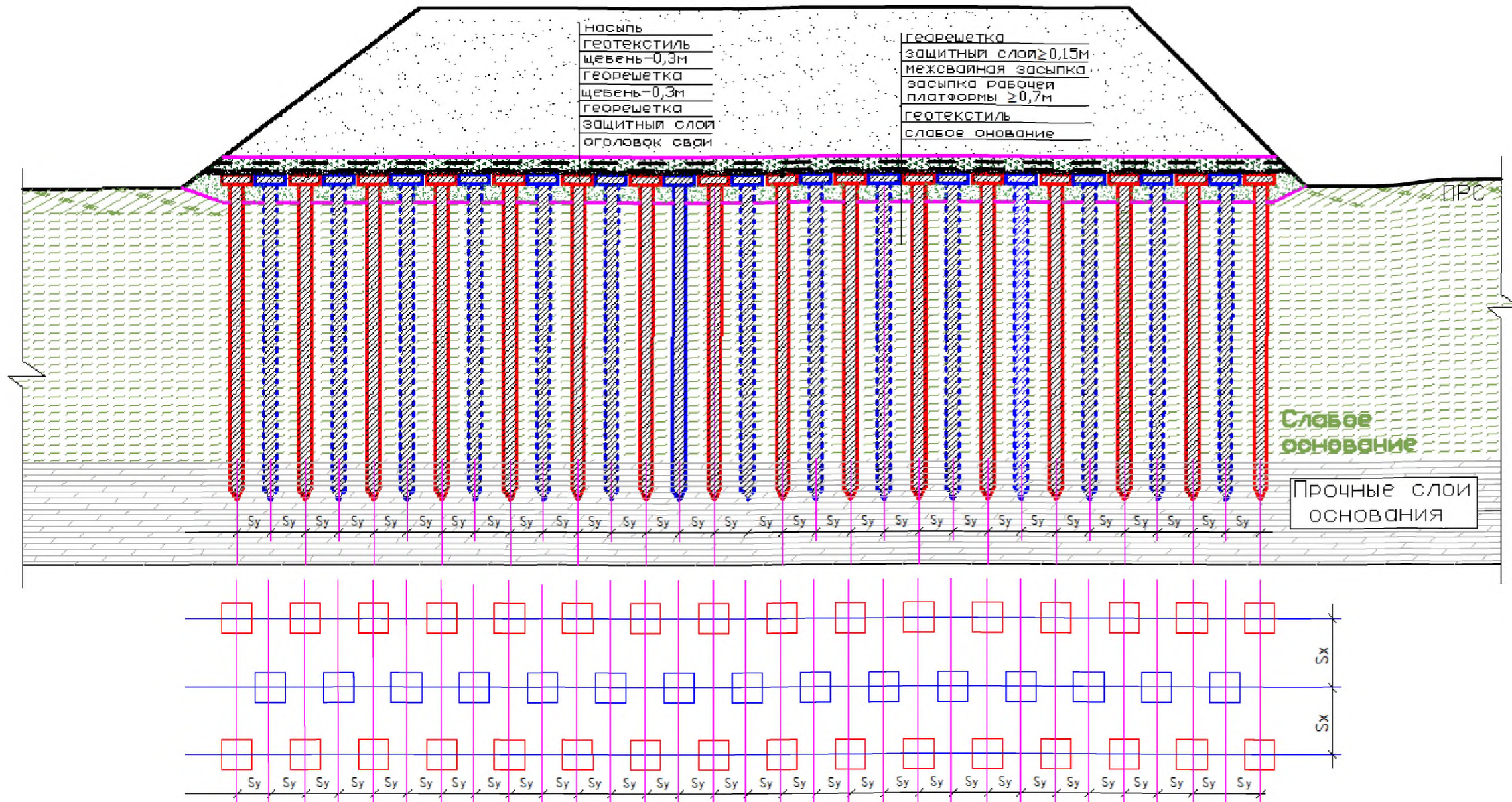
Рисунок А.8 Гибкий ростверк из двух слоев георешетки со щебнем на железобетонных сваях с оголовками (с размещением свай по треугольной сетке в «шахматном порядке»)
