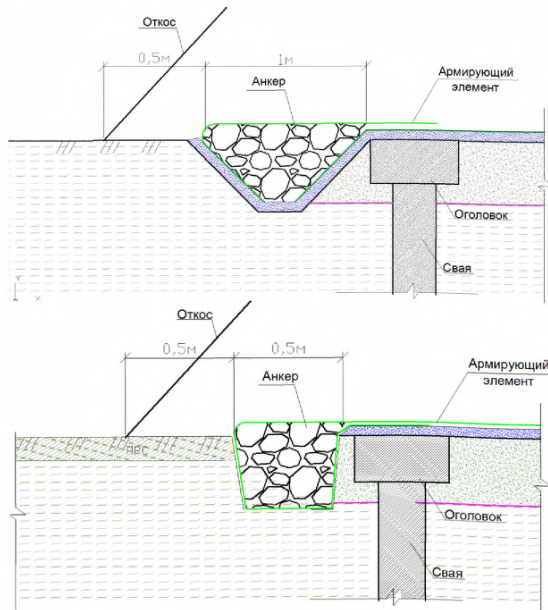
Рисунок 5 – Схемы конструктивных решений по анкерке армирующего элемента
