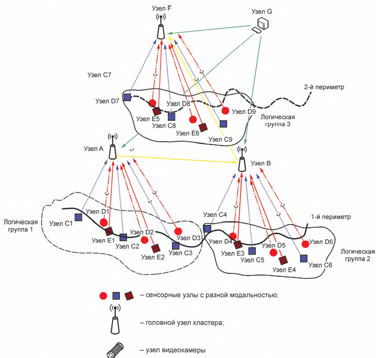
Рисунок В.1 — Отслеживание целей на основе расширенных служб, поддерживающих SIP
