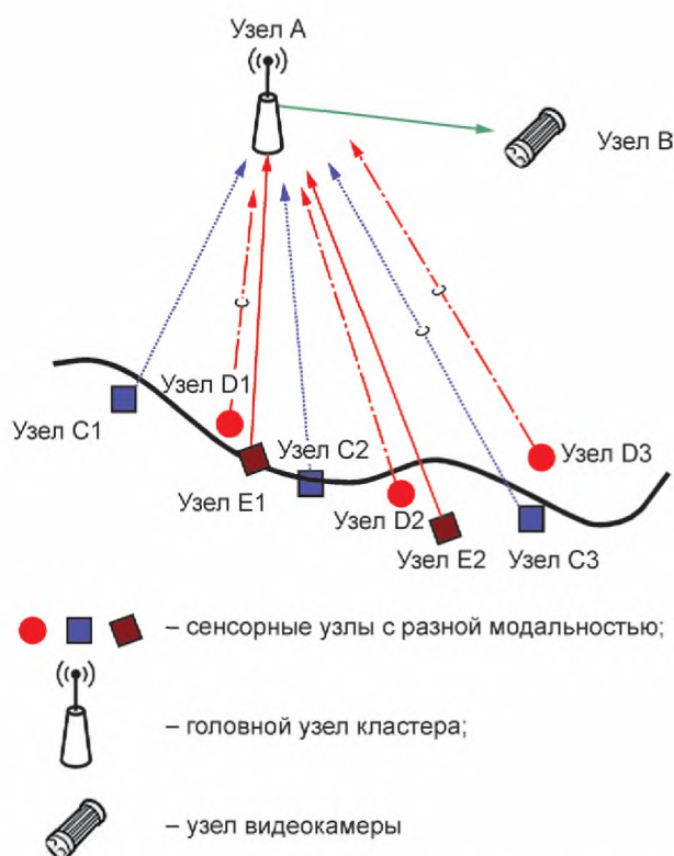
Рисунок А.1 — Обнаружение и распознавание целей на основе основных служб, поддерживающих СІР
