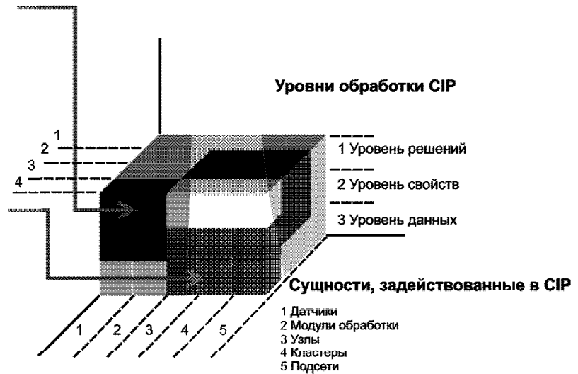
Рисунок 2 — Концептуальная модель СІР
