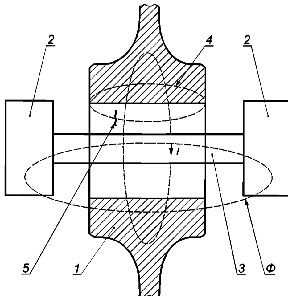
Рисунок В.1 — Схема полюсного намагничивания соленоидом колесного центра
