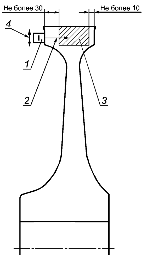
1 — прямой ПЭП; 2 — направление прозвучивания; 3 — зона контроля колесного центра; 4 — направление смещения ПЭП при сканировании
