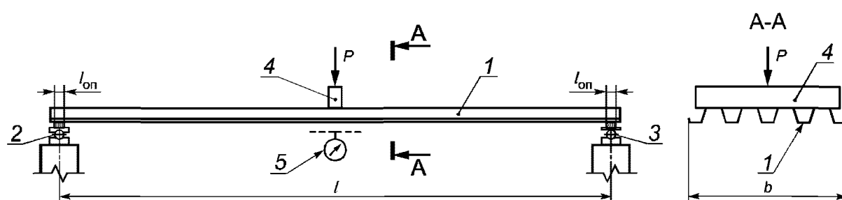
1 — испытываемый образец; 2 — неподвижная опора станда; 3 — подвижная опора станда; 4 — поперечная распределительная балка; 5 — индикатор прогиба
