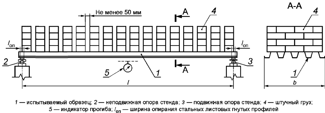
Рисунок 7 — Схема испытательного стэнда по схеме 1 — однопролетная балка
