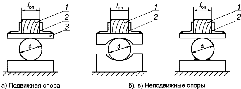
1 — деревянный брусок; 2 — стальной уголок; 3 — стальная пластина
