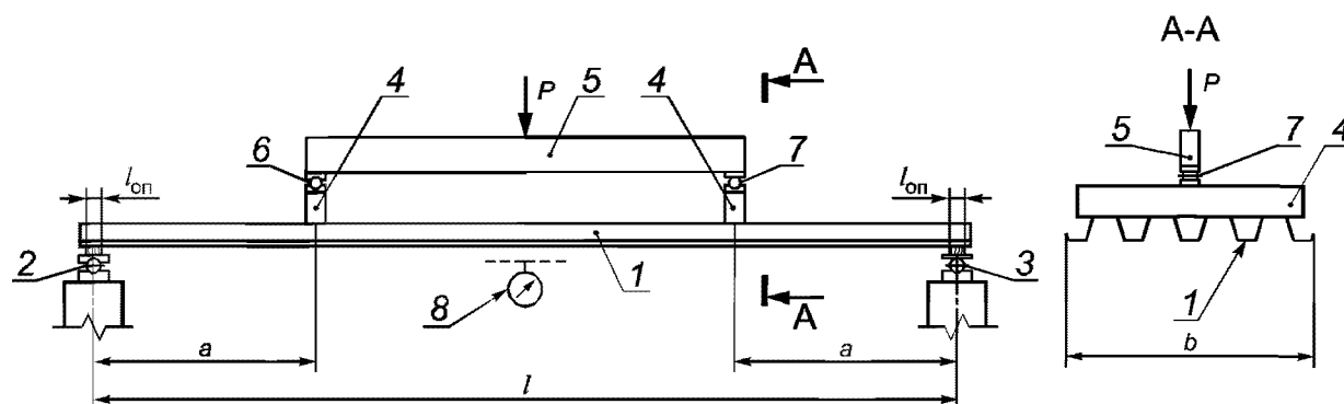
1 — испытываемый образец; 2 — неподвижная опора станда; 3 — подвижная опора станда; 4 — поперечная распределительная балка; 5 — траверса; 6 — неподвижная опора траверсы; 7 — подвижная опора траверсы; 8 — индикатор прогиба
