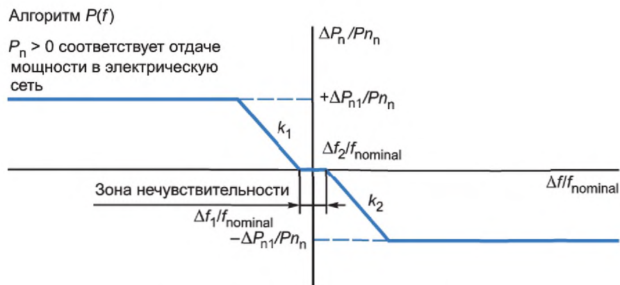
Рисунок 6 — Пример алгоритма P(f)
