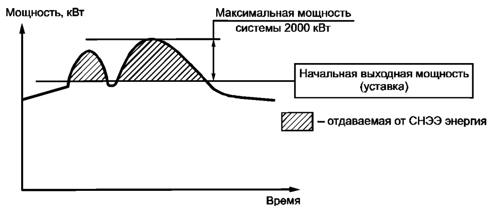
Рисунок 9 — Пример покрытия пиковых нагрузок
