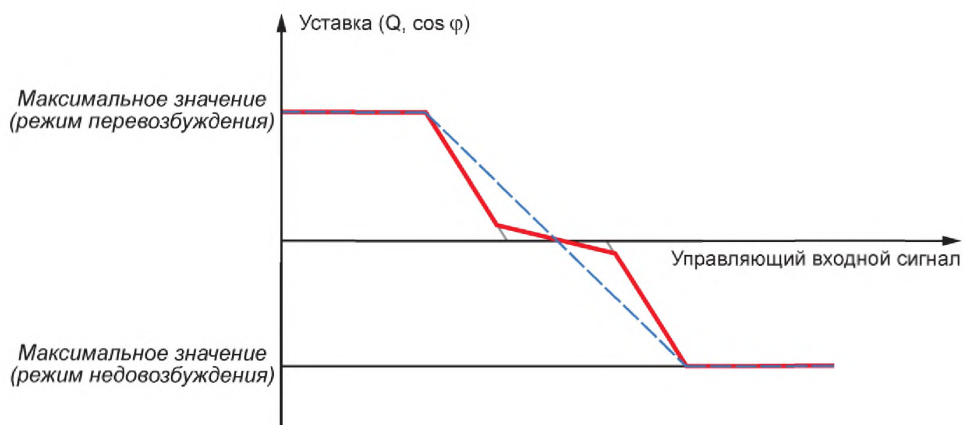
Рисунок 10 — Пример типовой характеристики регулирования [3], [4]
