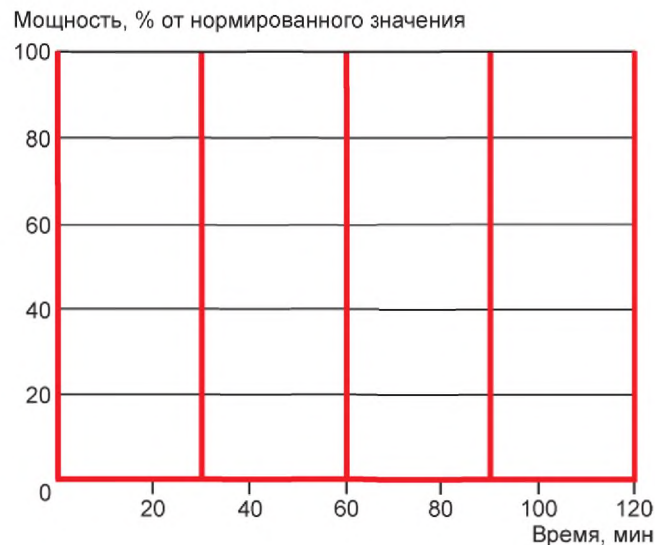
Рисунок А.1 — Пример рабочего цикла приложения резервирования функции первичного регулирования частоты сети [5]
