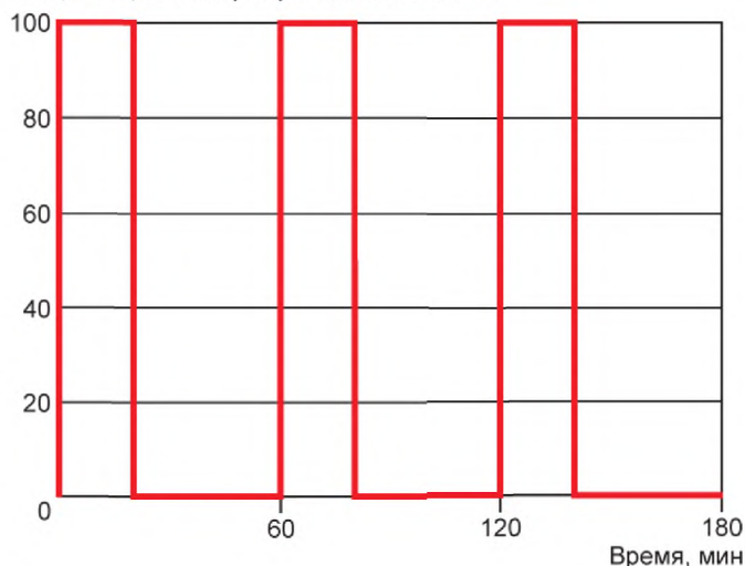
Рисунок А.2 — Пример рабочего цикла приложения резервирования функции вторичного регулирования частоты сети [4]
