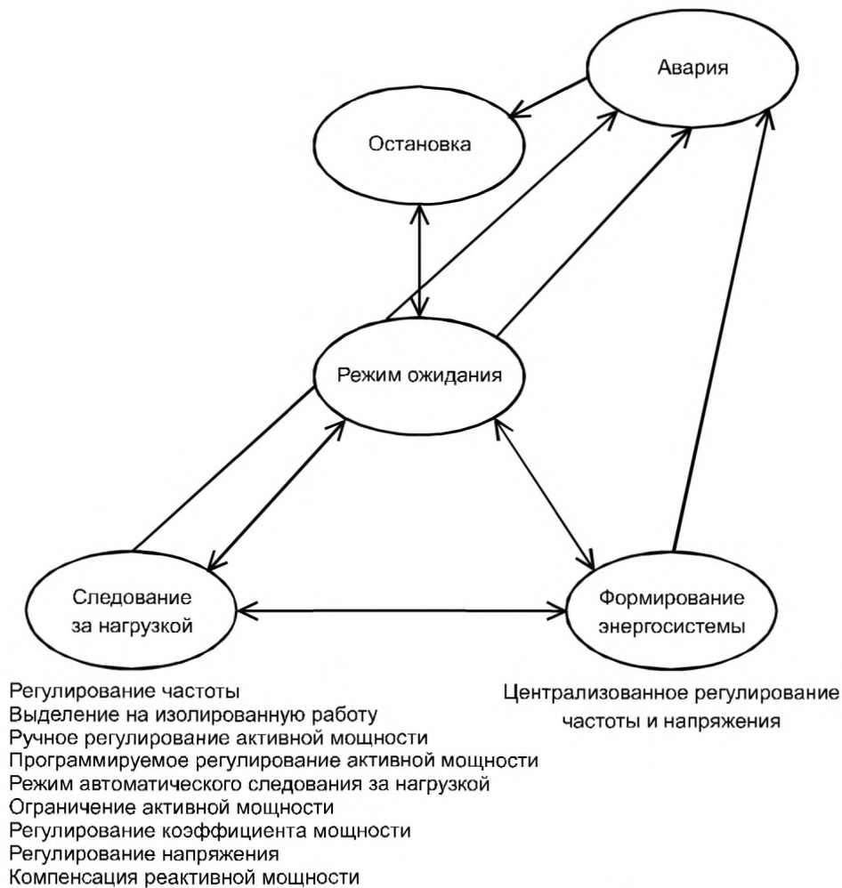
Рисунок 5 — Пример рабочих режимов СНЭЭ
