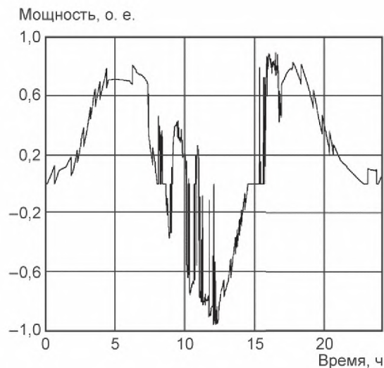
Рисунок А.7 — Пример изменения реактивной мощности СНЭЭ в ТПН [5]
