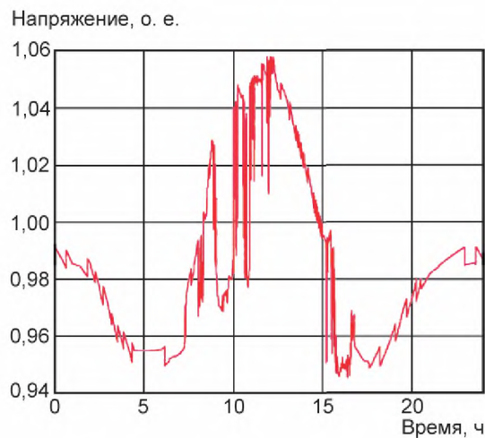
Рисунок А.6 — Пример изменения напряжения в ТПН [5]
