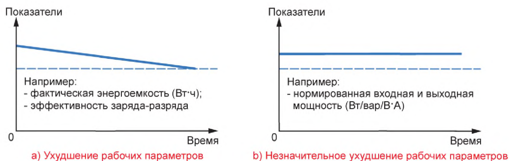
Рисунок 3 — Ухудшение отдельных рабочих параметров СНЭЭ с течением времени
