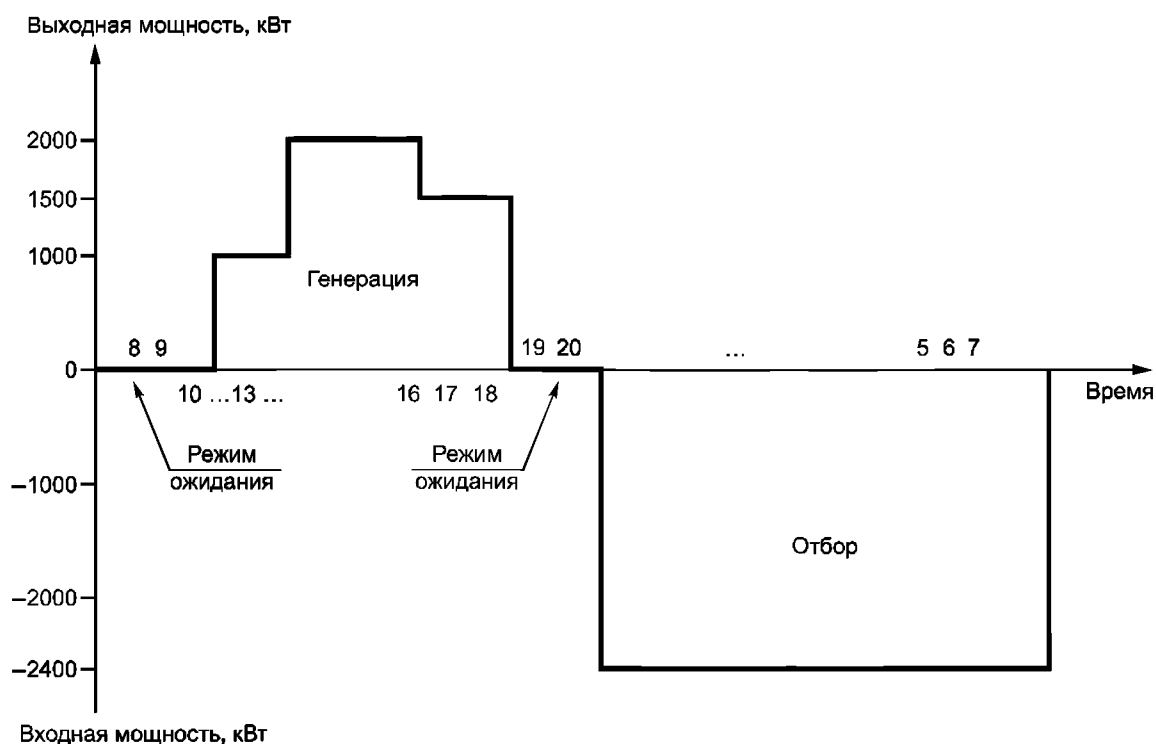
Рисунок 8 — Пример суточного рабочего графика в основной ТПН
