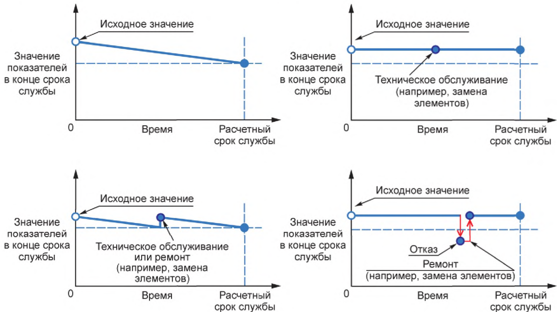
Рисунок 4 — Факторы, учитываемые при определении расчетного срока службы СНЭЭ
