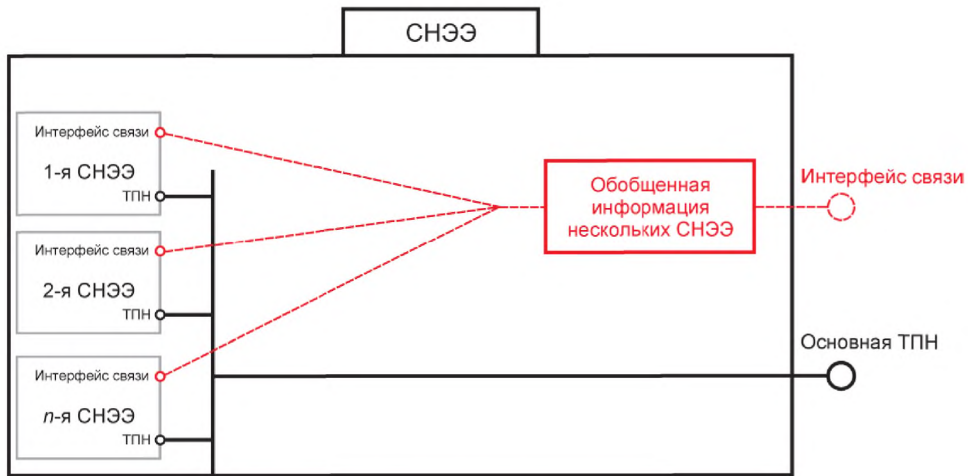
Рисунок 12 — Совокупность нескольких СНЭЭ, подсоединенных к одной ТПН
