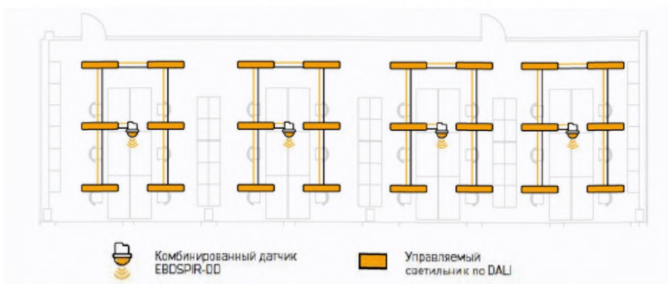
б) Средний сегмент – автоматическое управление
