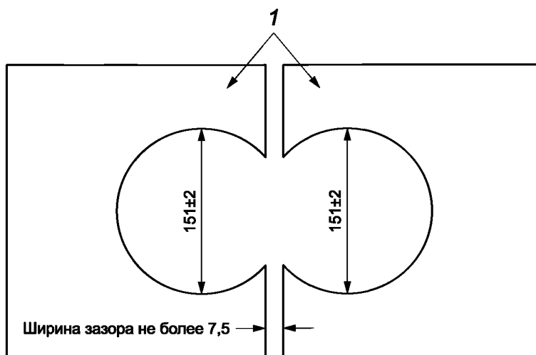
1 — части формы для установки образцов
