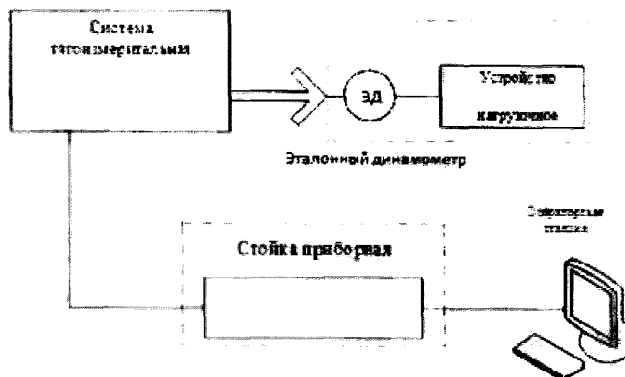
Рисунок 7 – Схема поверки ИК силы от тяги двигателя
