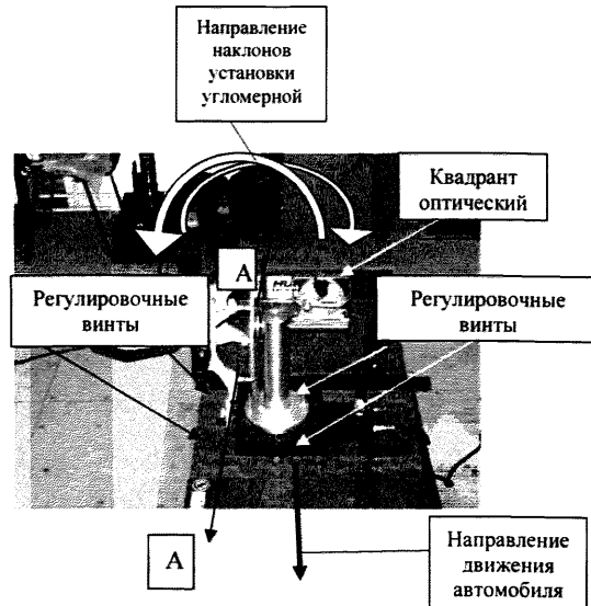
Рисунок 2 - Схема измерений углов развала колес
