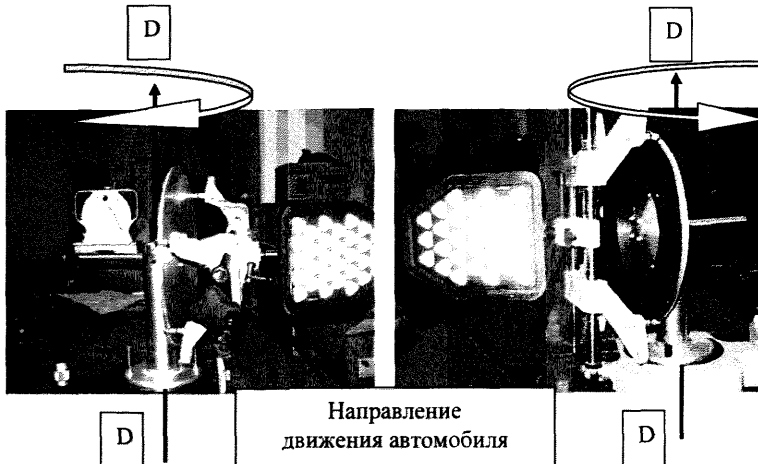
Рисунок 3 - Схема измерений углов индивидуального схождения колес
